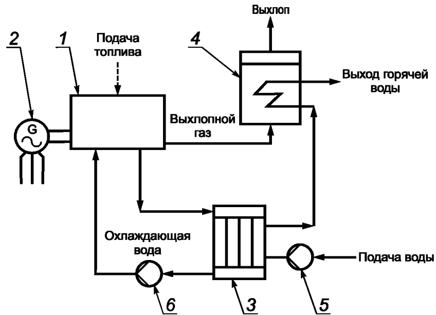
1 — закрытый поршневой двигатель внутреннего сгорания (бензиновый, дизельный); 2 — электрогенератор; 3 — низкотемпературный теплообменник; 4 — высокотемпературный теплообменник; 5 — насос горячей воды; 6 — насос охлаждающей воды
