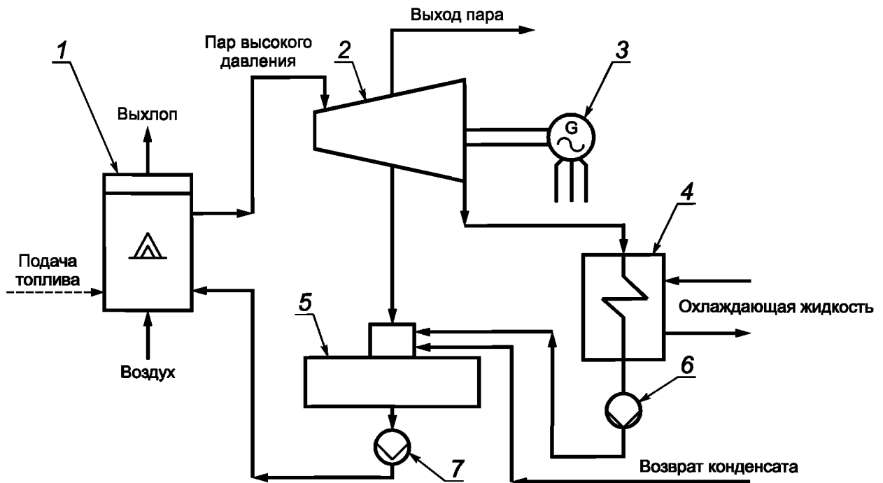
1 — традиционный парогенератор; 2 — паровая турбина; 3 — электрогенератор; 4 — конденсатор; 5 — водонагреватель; 6 — водяной насос; 7 — подающий водяной насос
