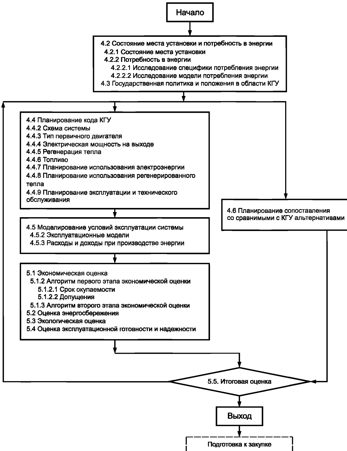
Рисунок 1 — Схема оценки КГУ
