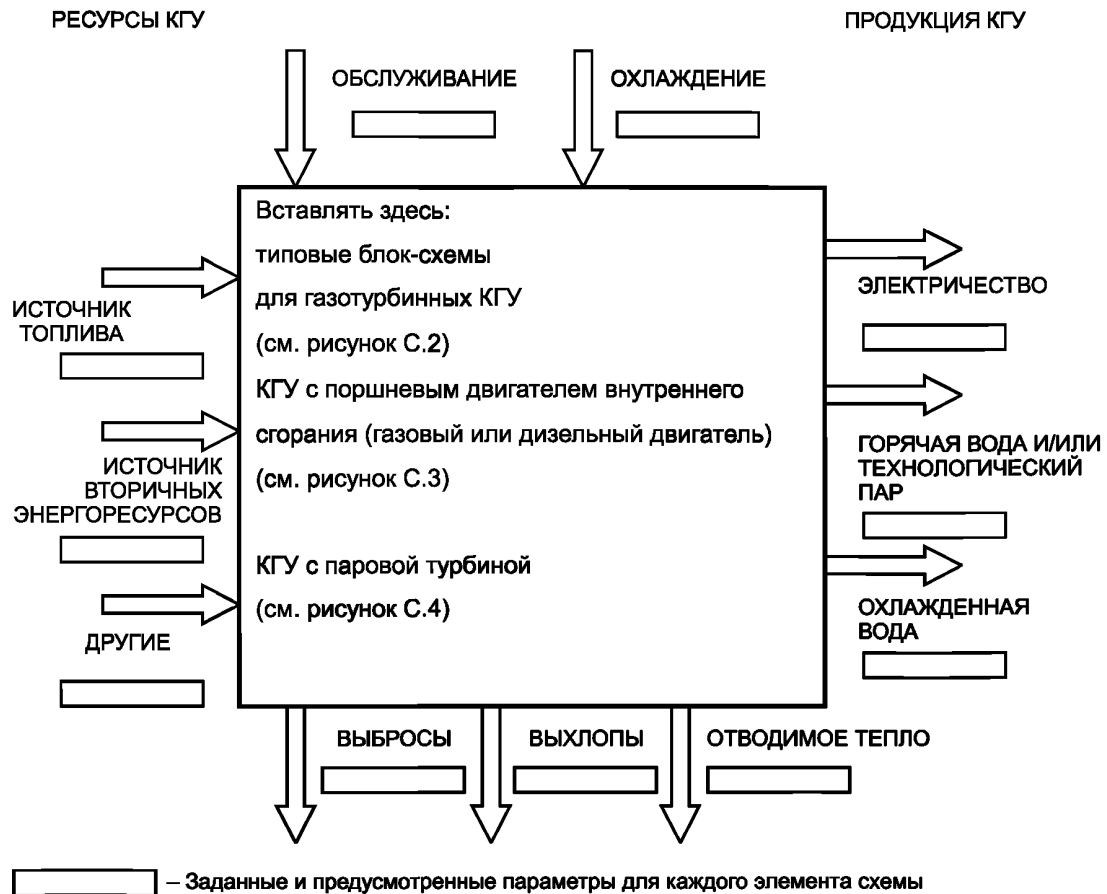
Рисунок С.1 — Типовая диаграмма КГУ
