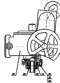
Рисунок Д.2 - Задвижка клиновая с выдвижным шпинделем с электроприводом (остальное - см. рисунок Д.1)
