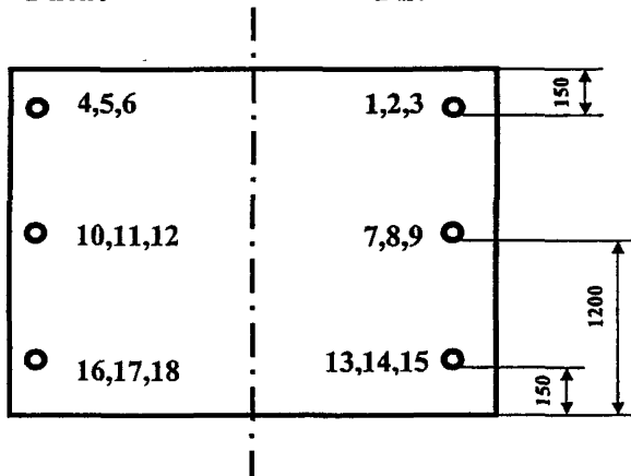
Рис. 2-2. Места установки датчиков температуры воздуха в помещениях площадью более 12 м 2
