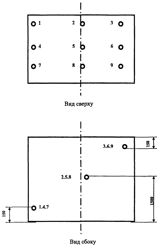
Рис. 2-1. Места установки датчиков температуры воздуха в помещениях площадью до 12 м 2 .
