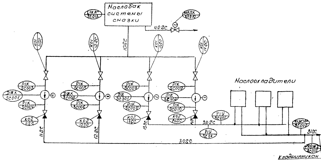
Локальная схема "SC" "основная система смазки".
