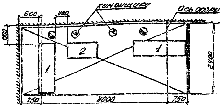
Рис. 3. Схема загрузки подмостей при ленточном замощивании
