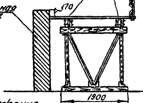
Рис.1. Установка подмоостей в рабочее положение
