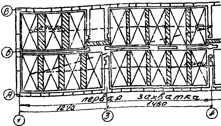
Рис. 2. Последовательность установки подмостей
