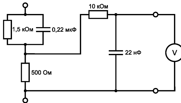
Рисунок 1 — Схема измерения тока прикосновения
