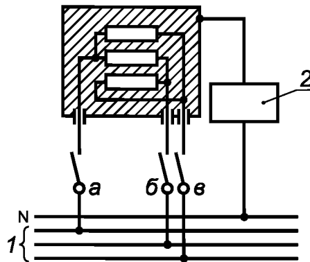
а, б, в — выключатели; N — нейтральный провод; 1 — трехфазное питание; 2 — схема по рисунку 1
