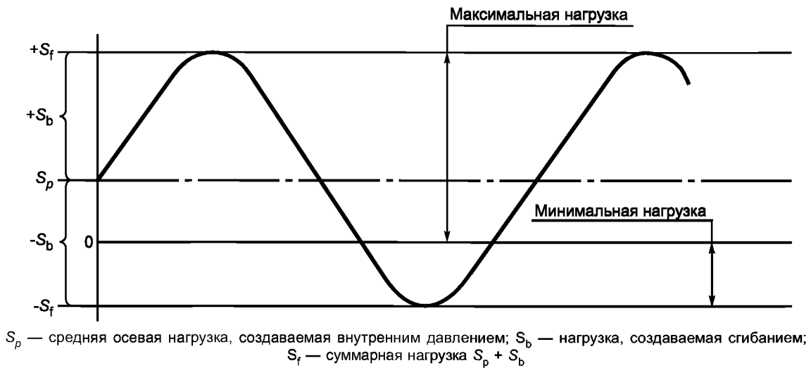
Рисунок 4 — Стандартный цикл переменной нагрузки при внутреннем давлении
