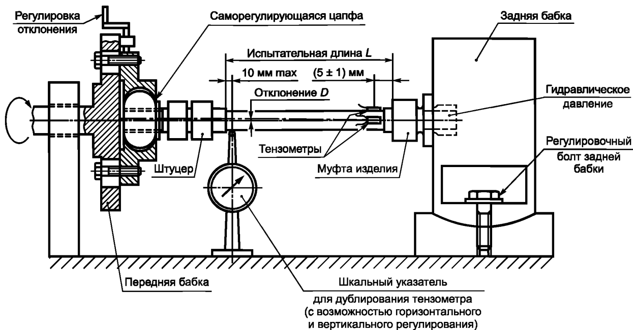
Рисунок 1 — Схема стандартного стенда для испытаний на изгиб
