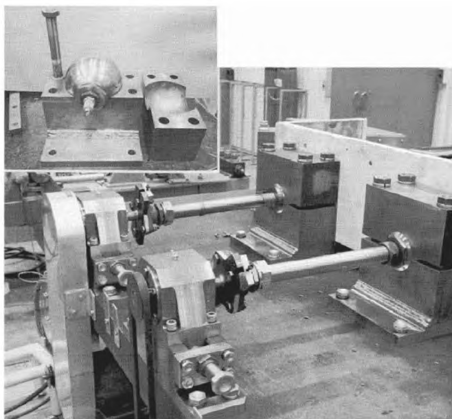
Рисунок 8 — Стенд для испытаний на изгиб трубопроводов диаметром не более DN 16
