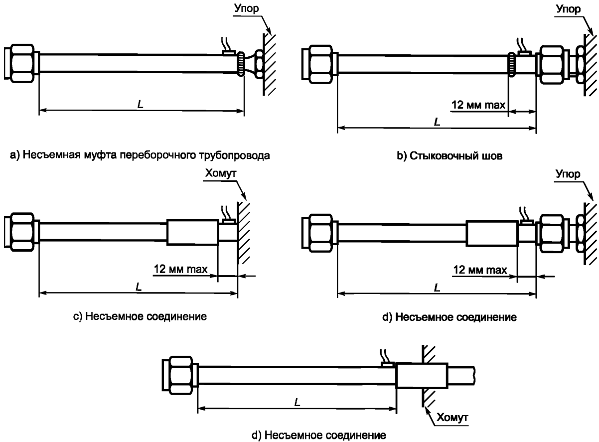
Рисунок 3 — Способы установки образцов с несъемной муфтой
