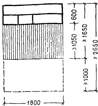
Рис. 25. Функциональная зона буфетной
