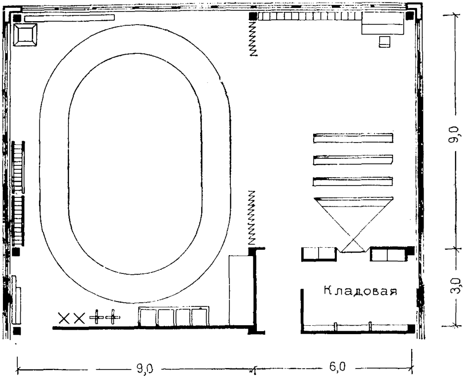
Рис. 29. Зал для музыкальных и гимнастических занятий площадью (100+50) м 2
