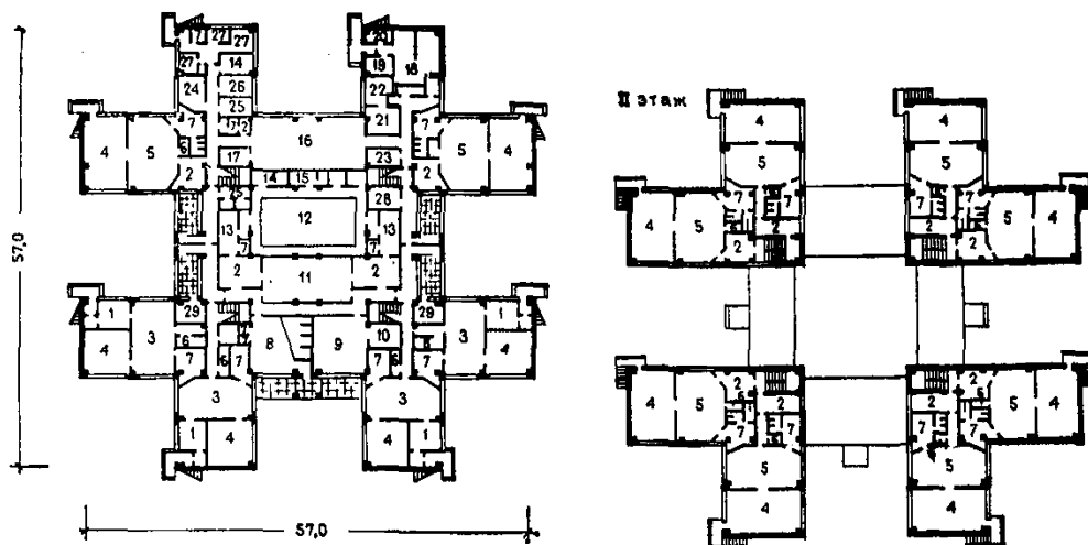
Рис. 37. Экспериментальный проект базового яслей-сада на 330 мест (шифр 76-008) (архит. Ф. Бабушкина, инж. Н. Максимова)
