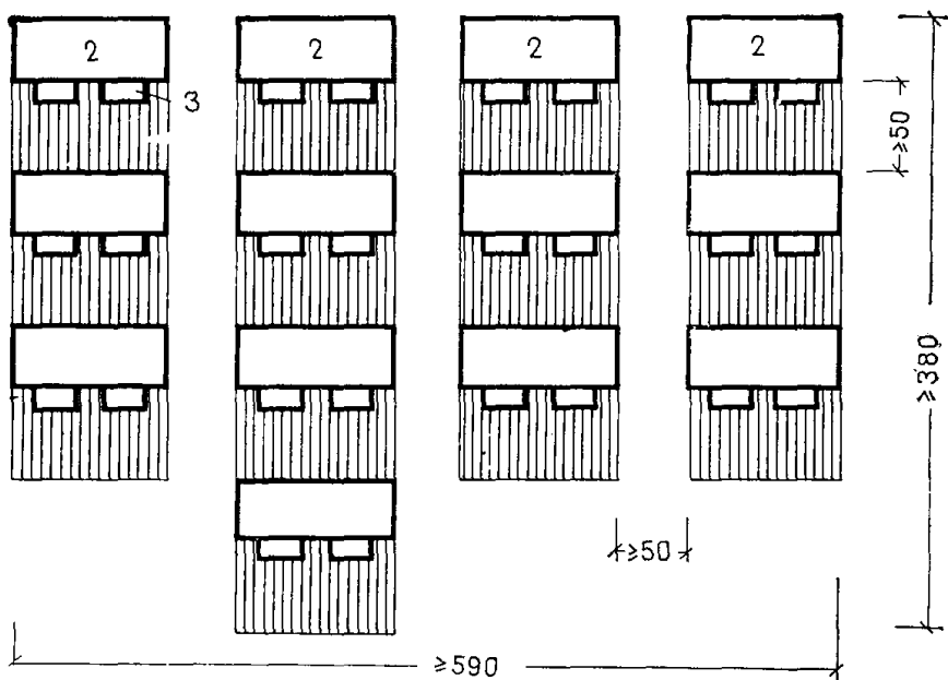
Рис. 23. Варианты размещения детских столов в игровых и групповых помещениях
