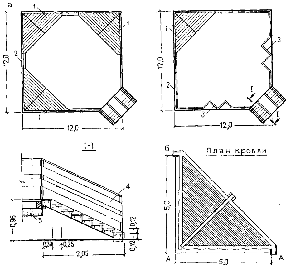
Рис. 6. Примеры решения групповых площадок-платформ для ясель-садов, проектируемых в районах с вечномёрзлыми грунтами
