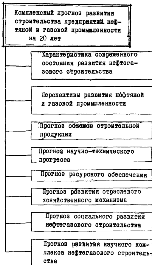
Рис.1. Структура Комплексного прогноза.
