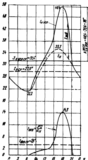
Рис. 9. Графическое определение амплитуды колебания температуры наружного воздуха с учетом солнечной радиации A_{\text{эксп}}^{\text{вн.}}_{\text{сол.}}
