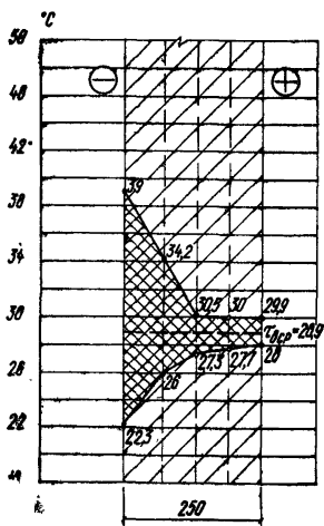
Рис. 8. Колебания температур в толще стены
