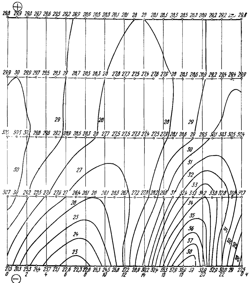
Рис. 7. Термоизоплеты стены
