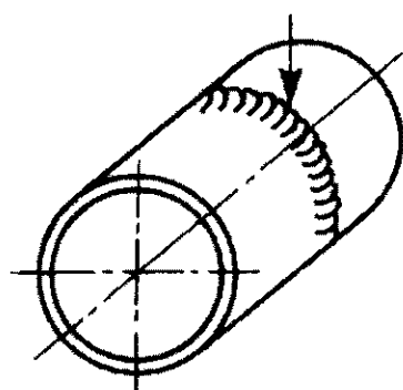
PA: Нижнее положение труба: поворачивается ось: горизонтальная
