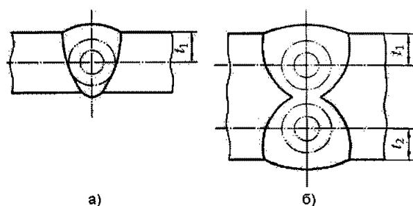
Рис. 6.4.4.1-5 Схема вырезки продольных цилиндрических образцов на растяжение:
