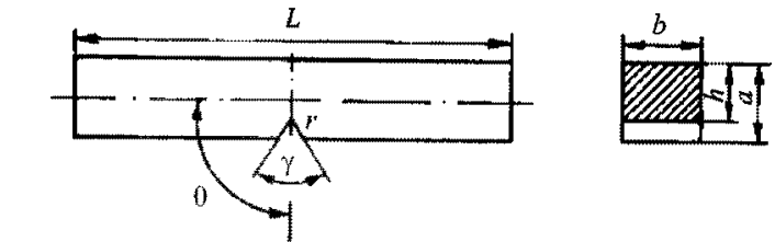
Рис. 6.4.4.2-3 Образец с продольным швом для испытаний на статический изгиб разнородных сварных соединений: А и В — части пробы из стали различных классов или категорий; L \approx 9a + D — для метода а) или L \approx 11a — для метода б); L — длина образца; a = t ; b = (t_w + 20) мм для t \leq 20 мм и b = (t_w + 30) мм для t > 20 мм
