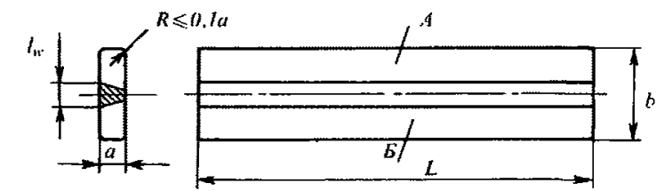
Рис. 6.4.4.2-3 Образец с продольным швом для испытаний на статический изгиб разнородных сварных соединений: А и В — части пробы из стали различных классов или категорий; L \approx 9a + D — для метода а) или L \approx 11a — для метода б); L — длина образца; a = t ; b = (t_w + 20) мм для t \leq 20 мм и b = (t_w + 30) мм для t > 20 мм
