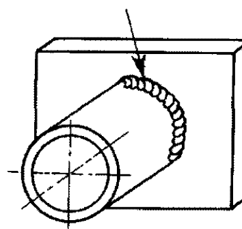
РВ: Горизонтально-вертикальное положение труба: поворачивается ось: горизонтальная
