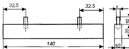
Пластина для фиксирования зазора
