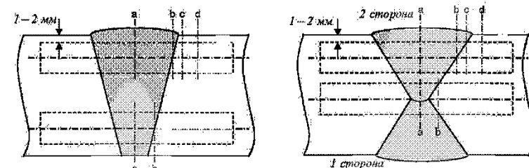
Рис. 6.4.4.4 Схема вырезки и расположения надреза на образцах для испытаний на ударный изгиб для технологических процессов сварки сталей высокой прочности:
