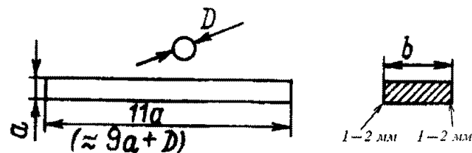
Рис. 6.4.4.2-1 Образцы для испытаний на статический изгиб: а) при t < 12 мм (образцы с растяжением корня и поверхности шва) a = t , b = 30 мм; б) при t \geq 20 мм (образцы на боковой изгиб) a = 10 мм, b = t ; в) при 12 \leq t < 20 допускается применение образцов типа а) или б); t — толщина металла испытуемой пробы
