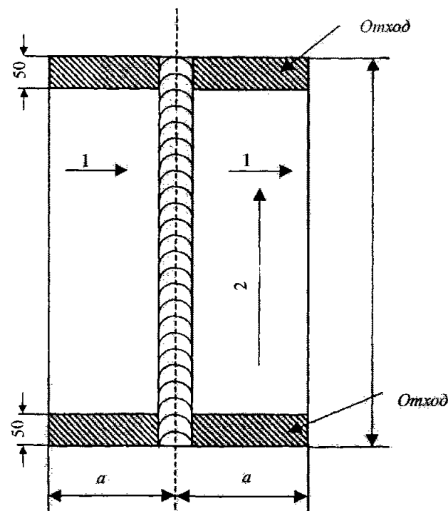
Рис. 6.3.1.2 Проба стыкового сварного соединения листов:
