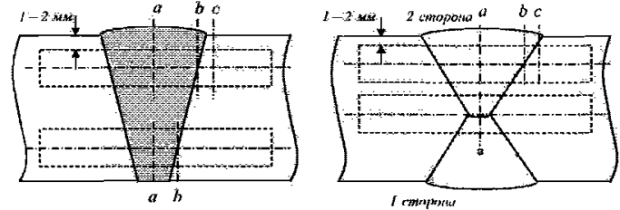
Рис. 6.4.4.4-2 Схема вырезки и расположения надреза на образцах для испытаний на ударный изгиб для технологических процессов сварки с погонной энергией \leq 50 кДж/см: а — надрез по центру шва (WM); б — надрез по линии сплавления (FL); с — надрез по ЗТВ на расстоянии 2 мм от линии сплавления (FL + 2)
