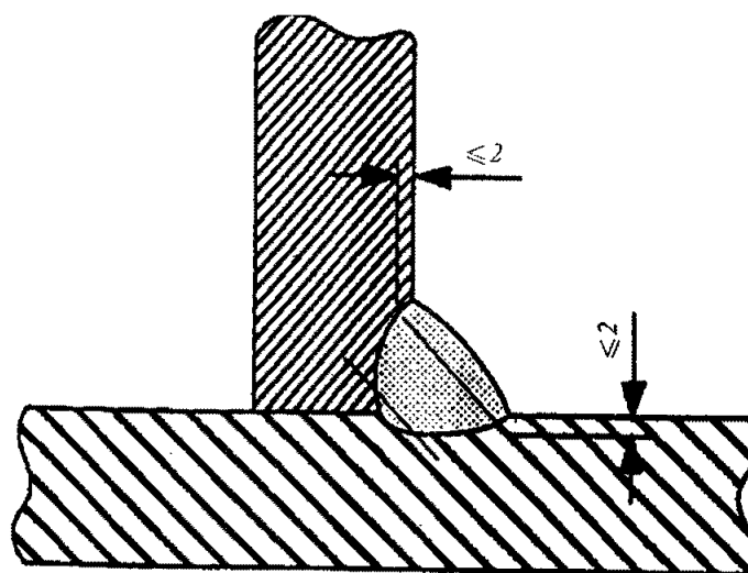
Рис. 6.4.4.5-5 Схема расположения линий замеров твердости в тавровых соединениях без разделки кромок, выполненных угловым швом
