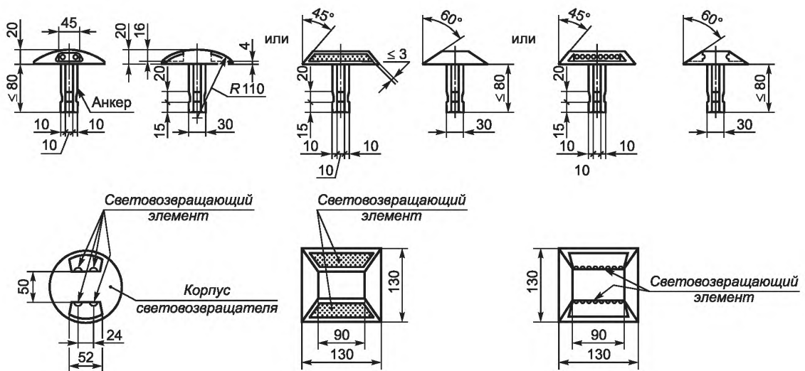
Рисунок Б.3 — Световозвращатели типа КДЗ
