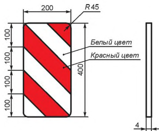
Рисунок Б.6 — Световозвращатель типа КД6
