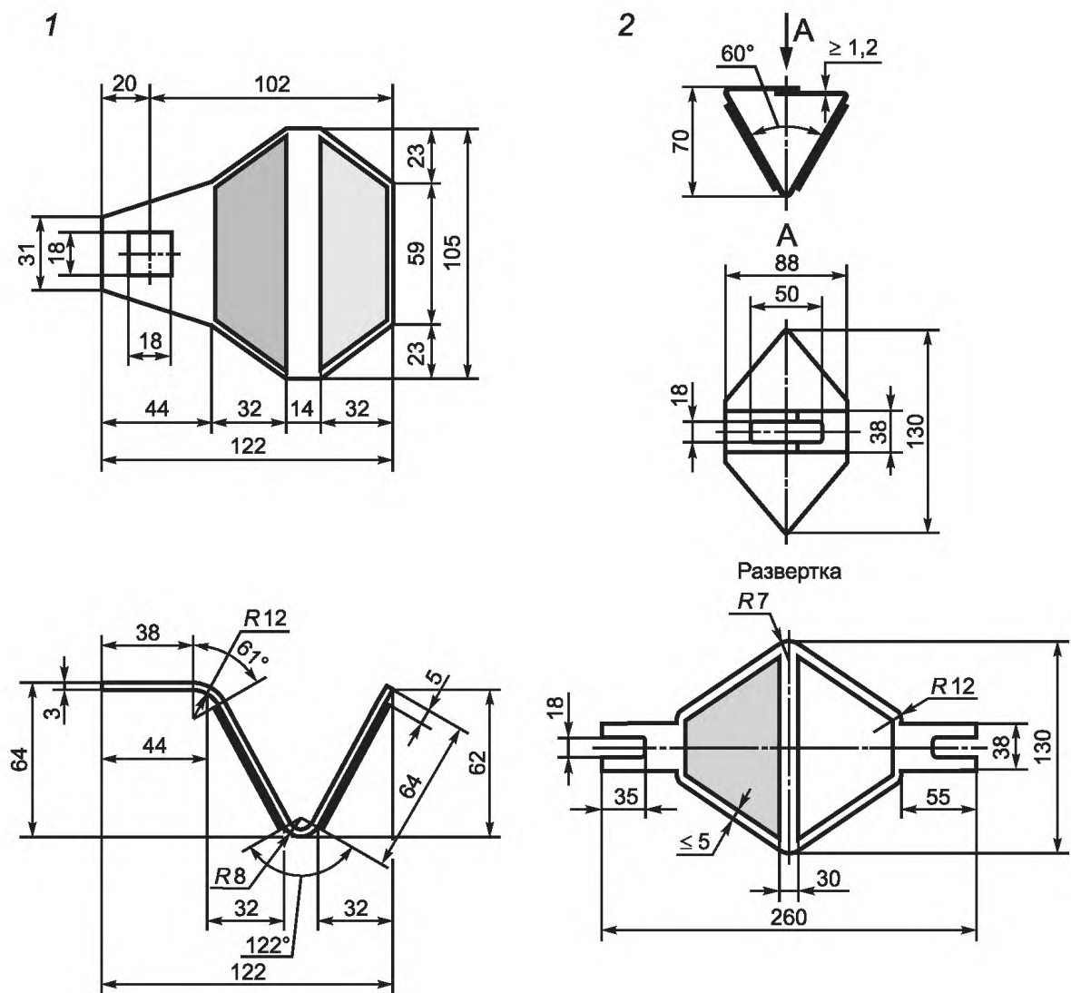
1 — вариант исполнения световозвращателя с консолью для крепления; 2 — вариант исполнения световозвращателя без консоли
