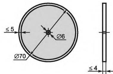
Рисунок Б.2 — Световозвращатель типа КД2
