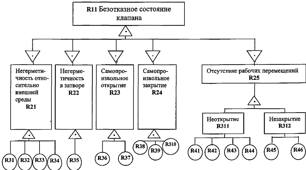
Рисунок И.1. Схема отказов клапана отсечного
