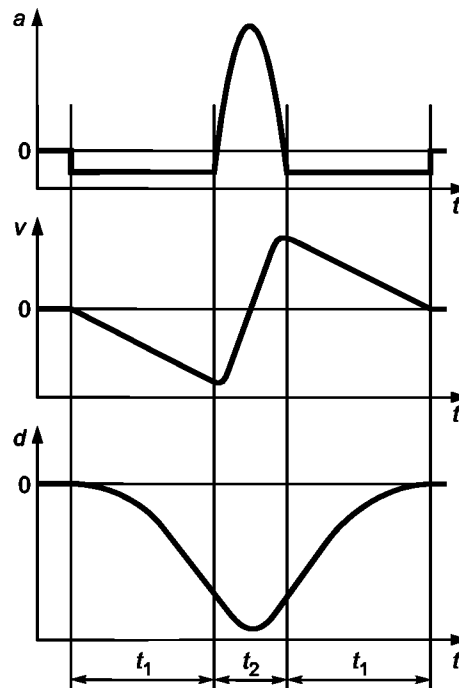
a — ускорение ударного импульса; v — скорость; d — перемещение; t — время; t_1 — длительность предударного (послеударного) импульса; t_2 — длительность импульса (основной части)
