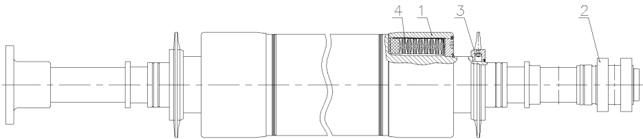
а)– Ротор турбогенератора ТГВ-25 (поз.4 рис.5.1а)
