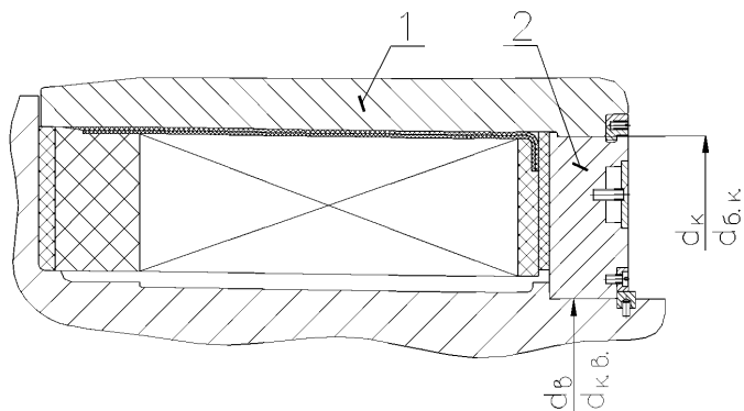
1 – бандажное кольцо; 2 – центрирующее кольцо. б)- Бандажный узел ротора ТВС–30, поз.1 рис. 7.1б
