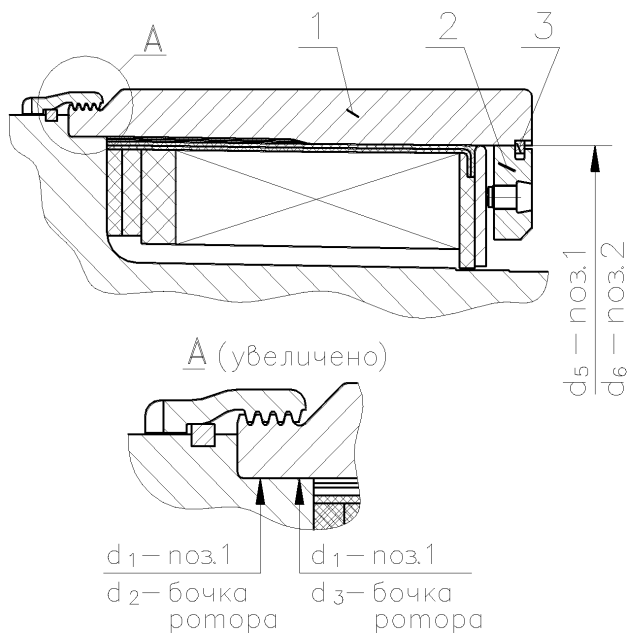
Рисунок 7.2 – Бандажный узел ротора консольного исполнения, поз.1 рисунок 7.1.
