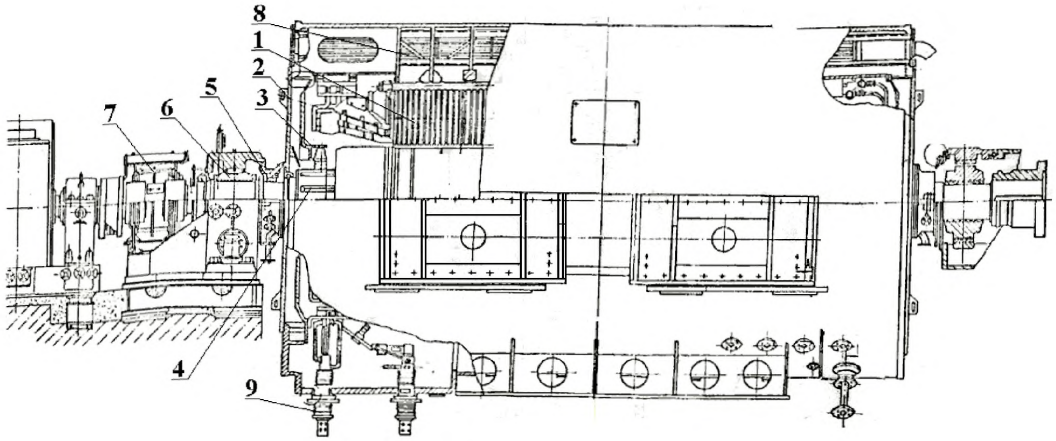
1 – статор; 2 – щит наружный; 3 – щит вентилятора; 4 – ротор; 5 – уплотнение вала ротора; 6 – подшипник; 7 – щеточный аппарат; 8 – газоохладитель; 9 – вывод концевой. Рисунок 5.1– Турбогенераторы ТВВ–160–2Е, ТВВ–220–2Е.
