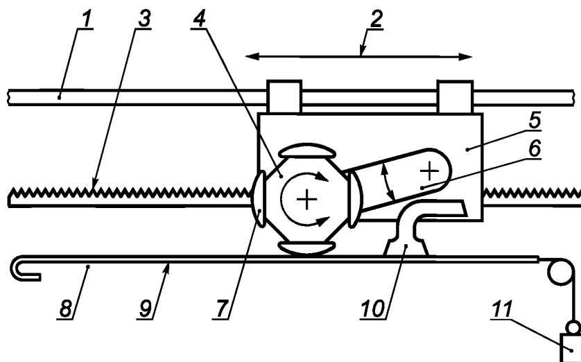
1 — направляющая планка; 2 — направление движения; 3 — зубчатая рейка; 4 — третрад; 5 — рама; 6 — кулиса; 7 — стопа; 8 — плоский столик для укладки проб; 9 — проба; 10 — пылесос; 11 — предварительная нагрузка
