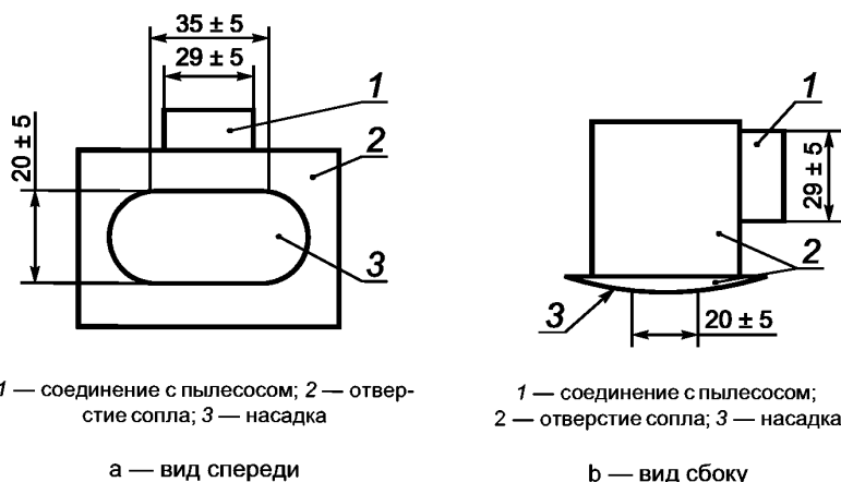
Рисунок 2 — Опора присоски
