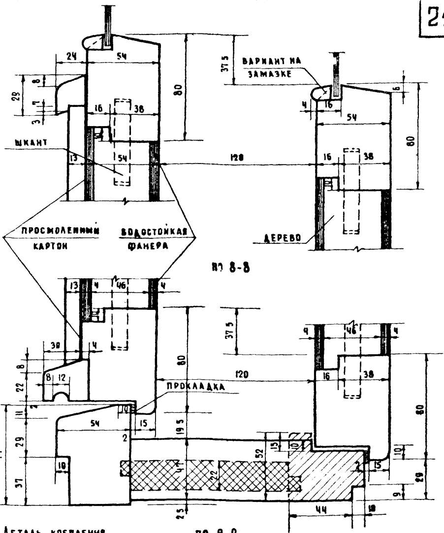
ДЕТАЛЬ КРЕПЛЕНИЯ У-ОБРАЗНОЙ ПРОКЛАДКИ. ГВОЗДИ Ф 10-10 ЧЕР 300-400 КЛЕЙ 88
