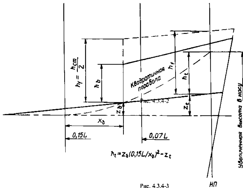
Рис. 4.3.4-3
