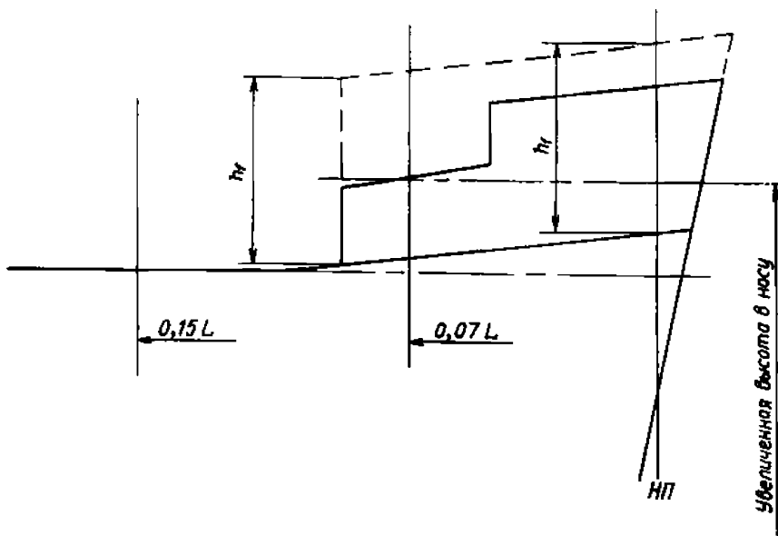
Рис. 4.3.4-3
