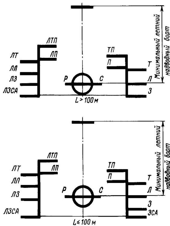
Рис. 5.2.3
