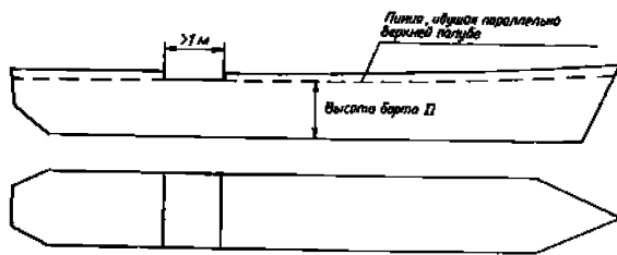
Рис. 1.2.1-2
