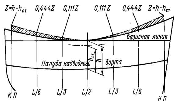
Рис. 4.3.1.5
