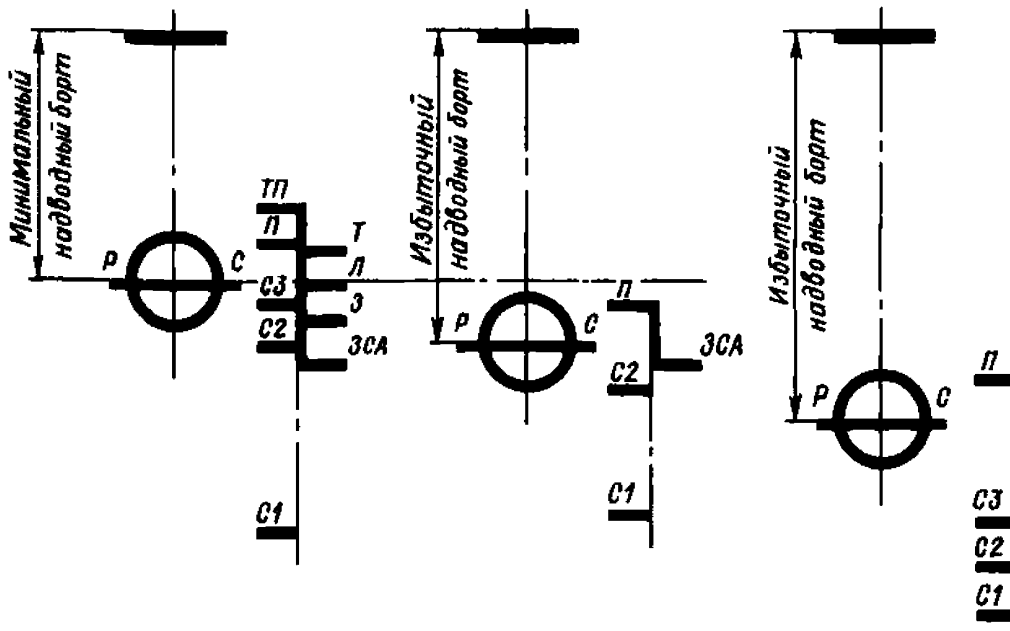
Рис. 2.2.6.2
