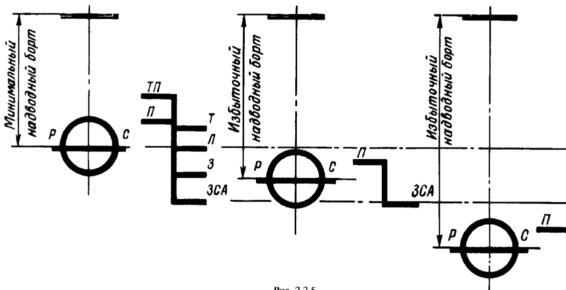
Рис. 2.2.5
