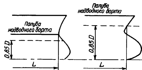
Рис. 1.2.1-1
