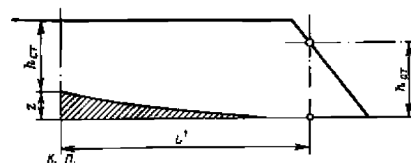
Рис. 4.3.4-1
