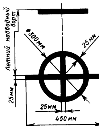
Рис. 6.2.2
