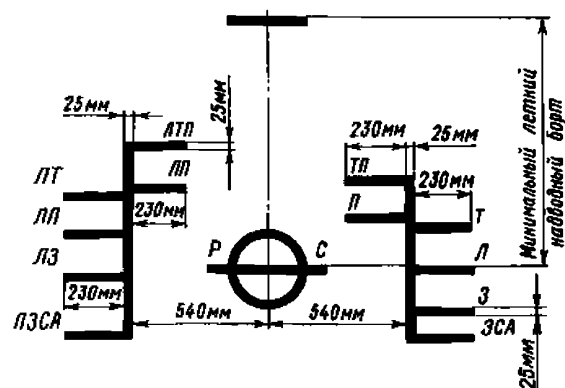
Рис. 2.2.1
