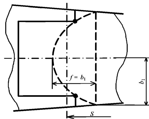
Рис. 4.2.2.3-2
