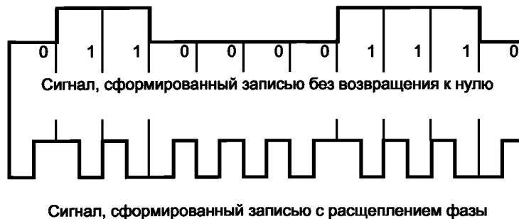
Рисунок В.2 — Кодирование с расщеплением фазы
