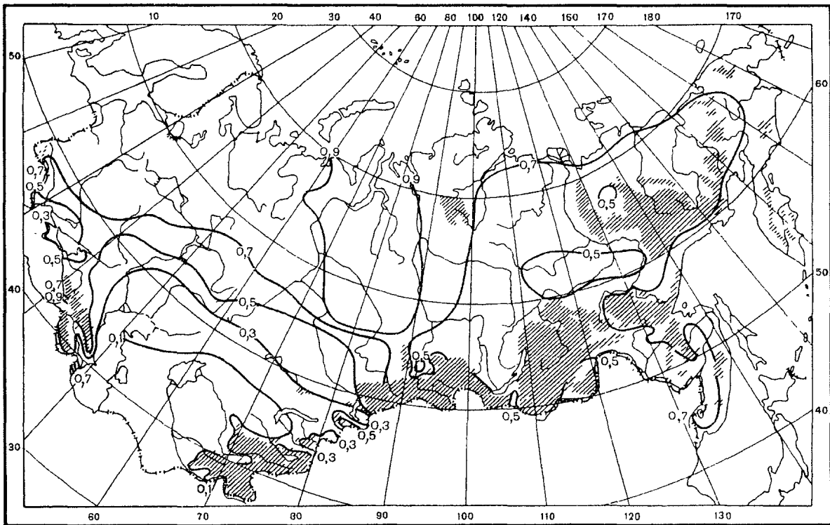
Рис. П2.16. Среднемесячное относительное испарение, E/E_0 . Июль
