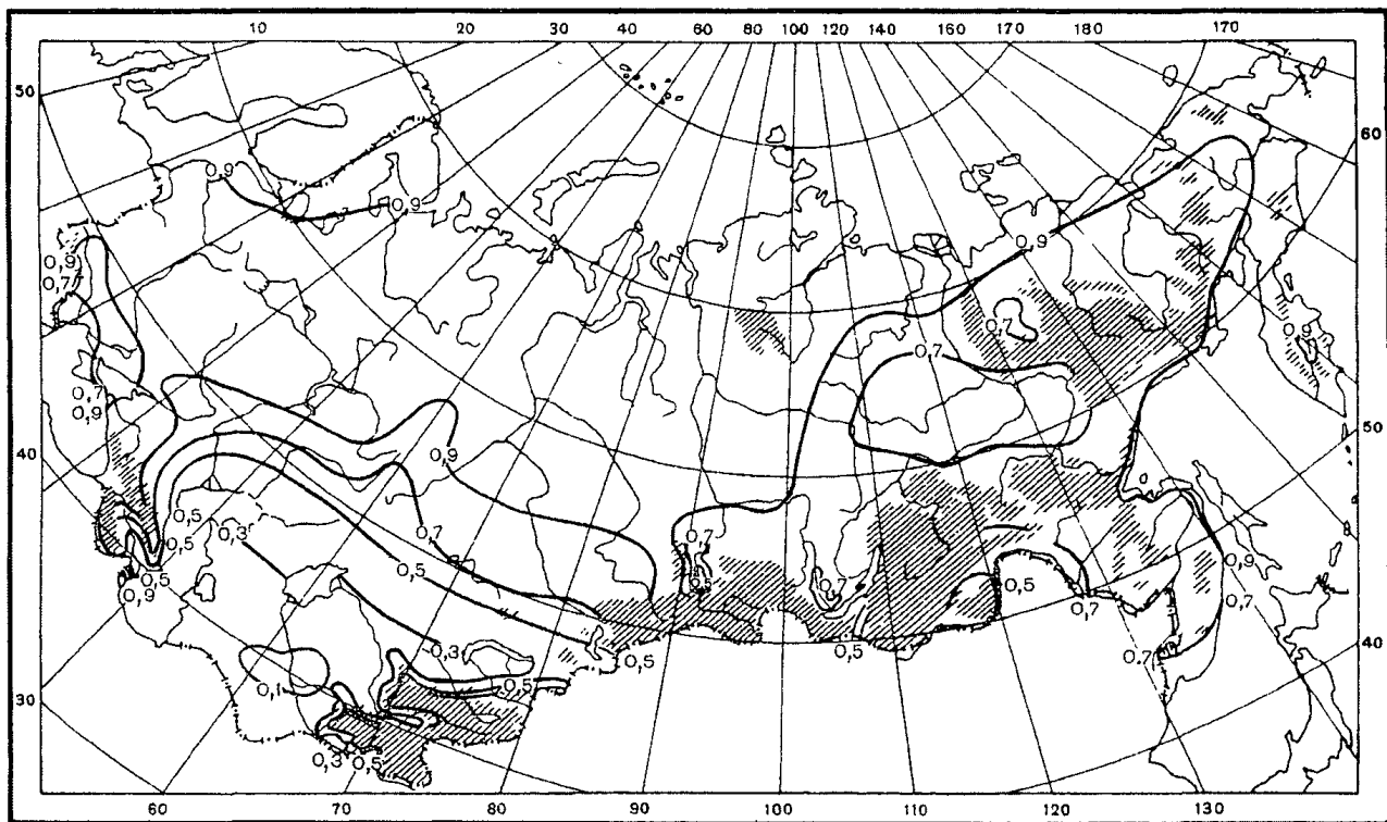
Рис. П2.14. Среднее месячное относительное испарение E/E_0 . Май ▨ – горные районы
