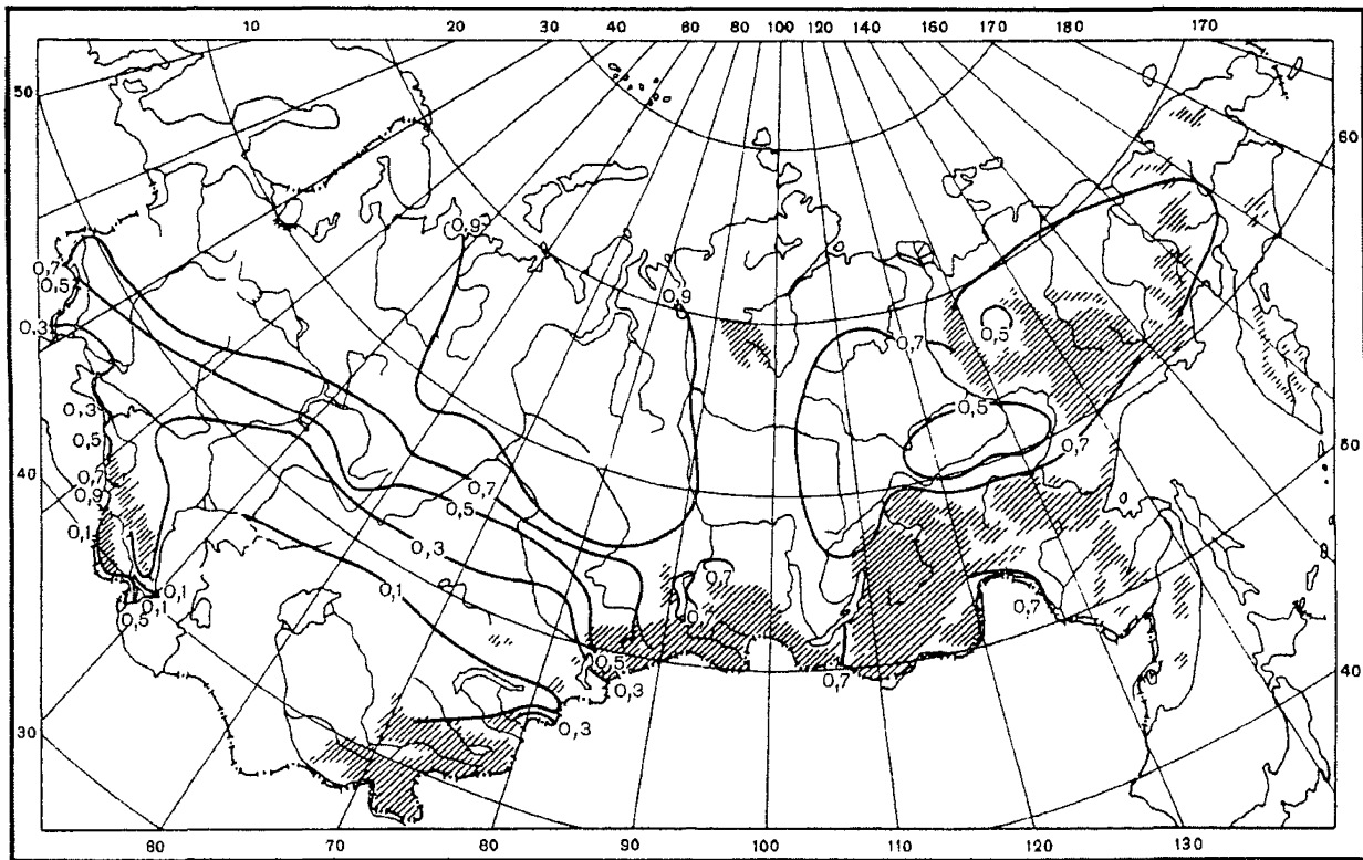
Рис. П2.18. Среднее месячное относительное испарение, E/E_0 . Сентябрь ▨ – горные районы
