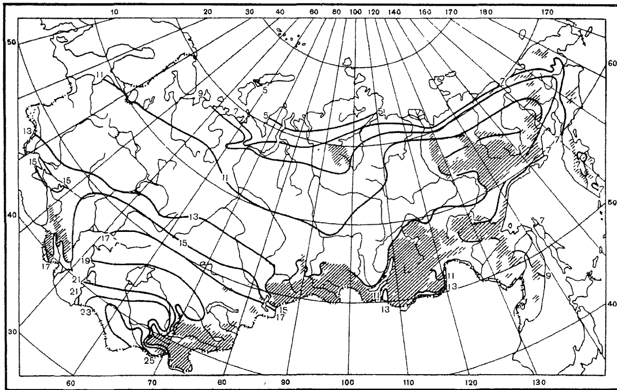
Рис. П2.8. Средняя месячная испаряемость, см. Июнь
