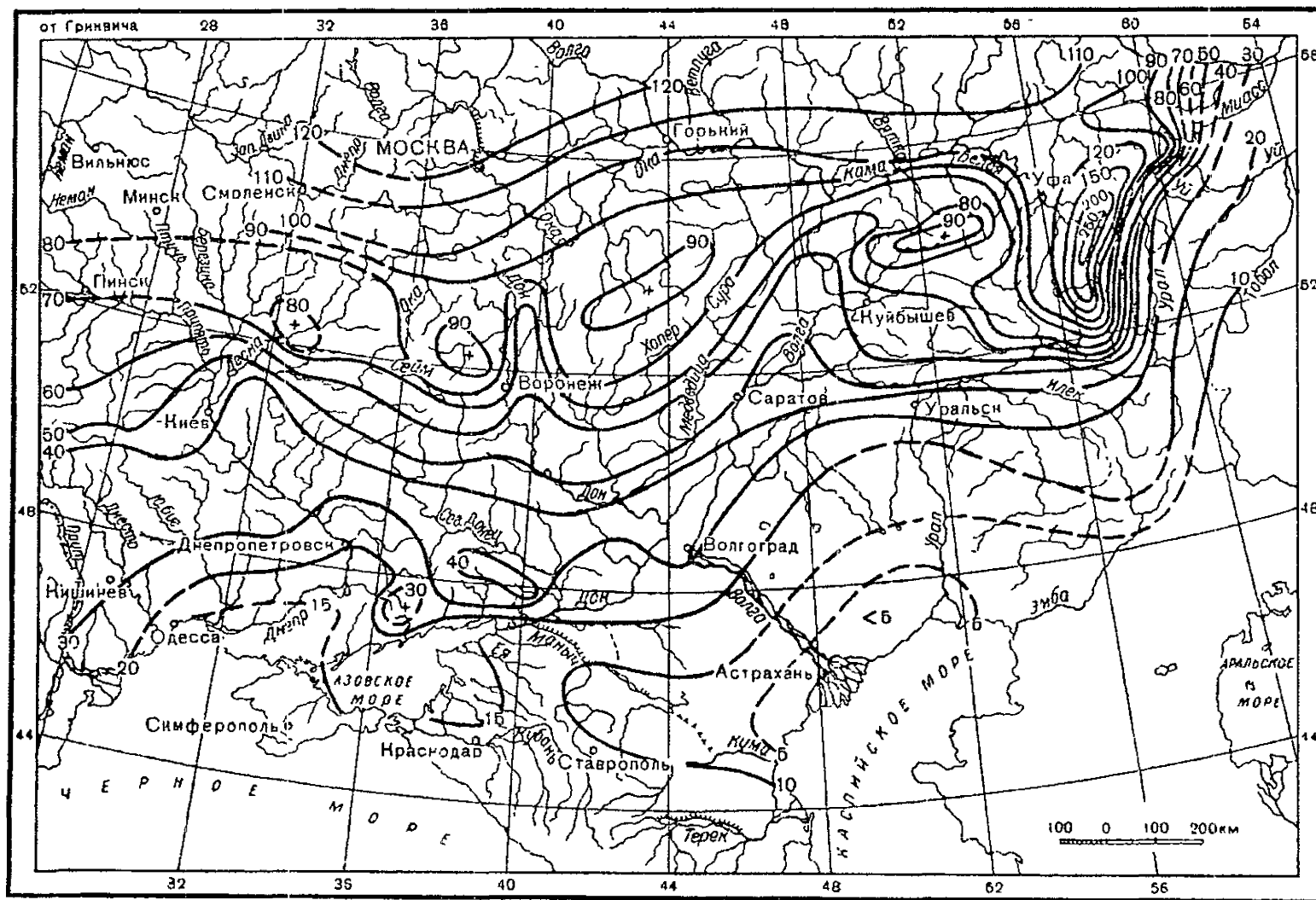
Рис. П2.21. Карта среднего слоя весеннего поверхностного стока рек (мм) лесостепной и степной зон (по К. П. Воскресенскому)
