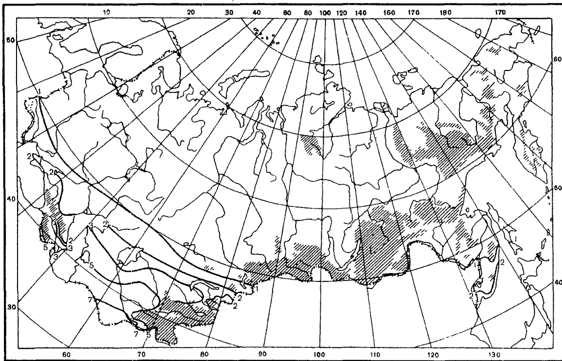
Рис. П2.13. Средняя месячная испаряемость, см. Ноябрь
