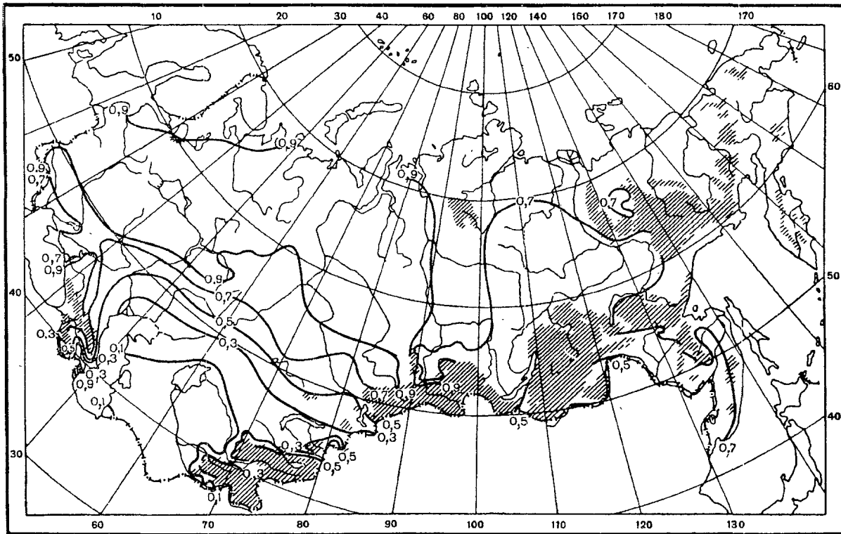
Рис. П2.15. Среднее месячное относительное испарение, E/E_0 . Июнь ▨ – горные районы
