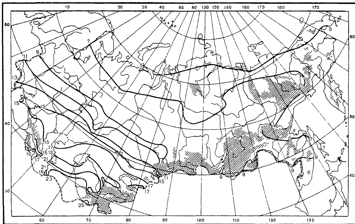
Рис. П2.10. Средняя месячная испаряемость, см Август ▨ – горные районы
