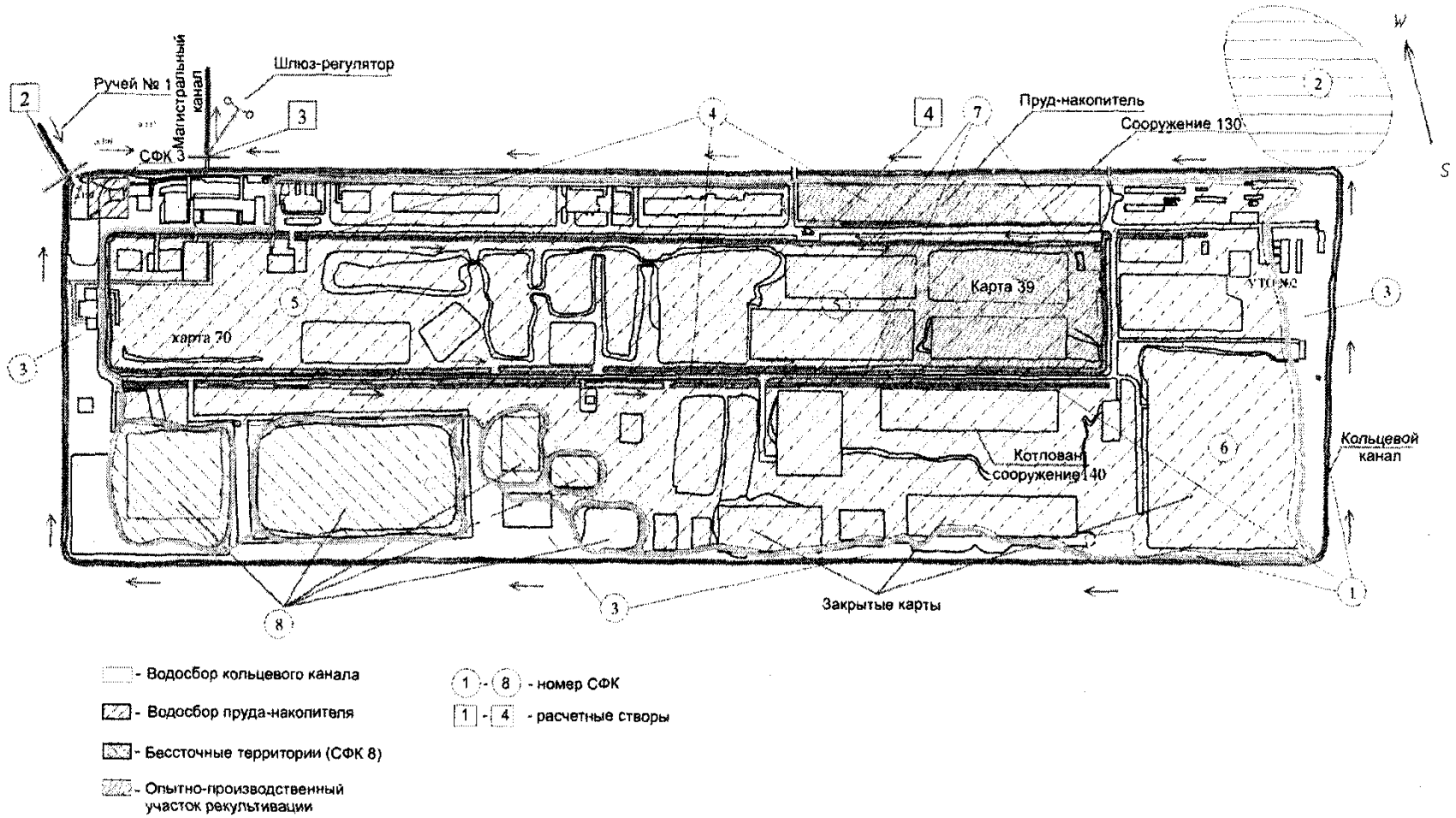
Рис. П.3.1. Схема территории полигона «Красный Бор»
