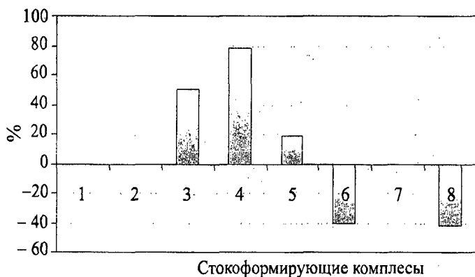
Рис. ПЗ.2. Изменение площадей стокоформирующих комплексов за период 1996 – 2004 гг. (в % от первоначальных)
