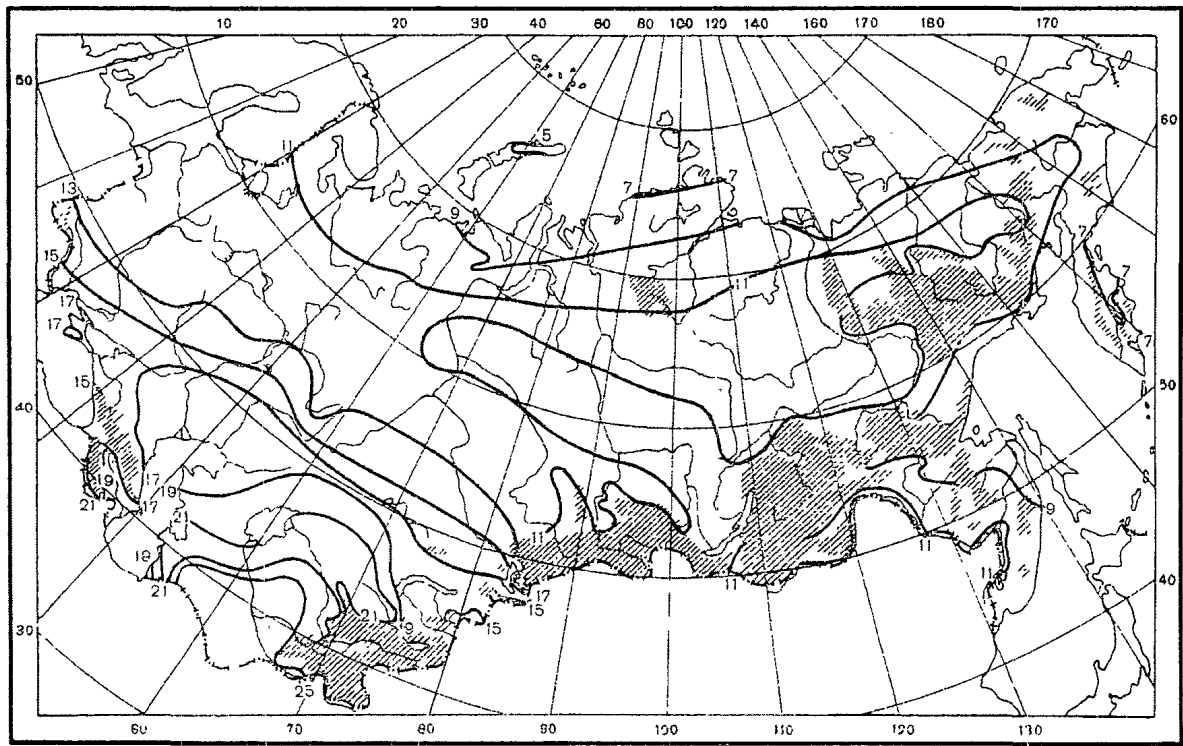
Рис. П2.9. Средняя месячная испаряемость, см. Июль ▨ – горные районы
