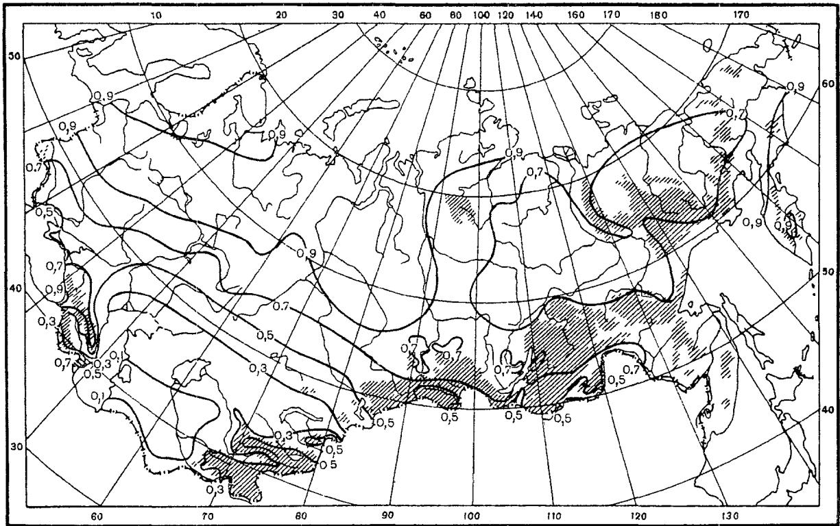
Рис. П2.3. Среднее годовое относительное испарение, E/E_0
