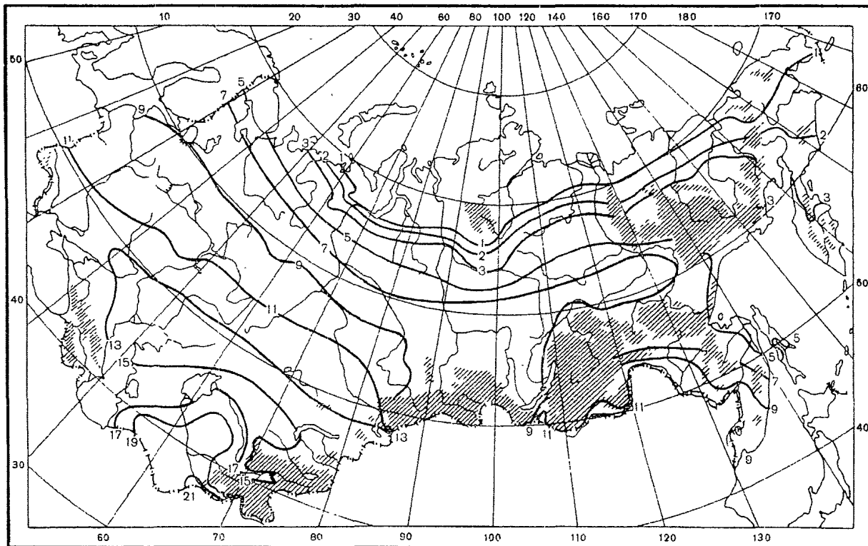
Рис. П2.7. Средняя месячная испаряемость, см. Май
