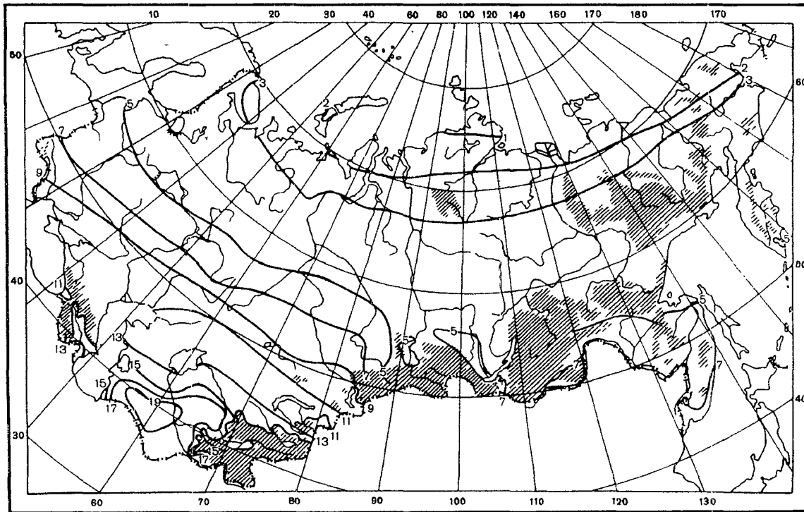
Рис. П2.11. Средняя месячная испаряемость, см. Сентябрь
