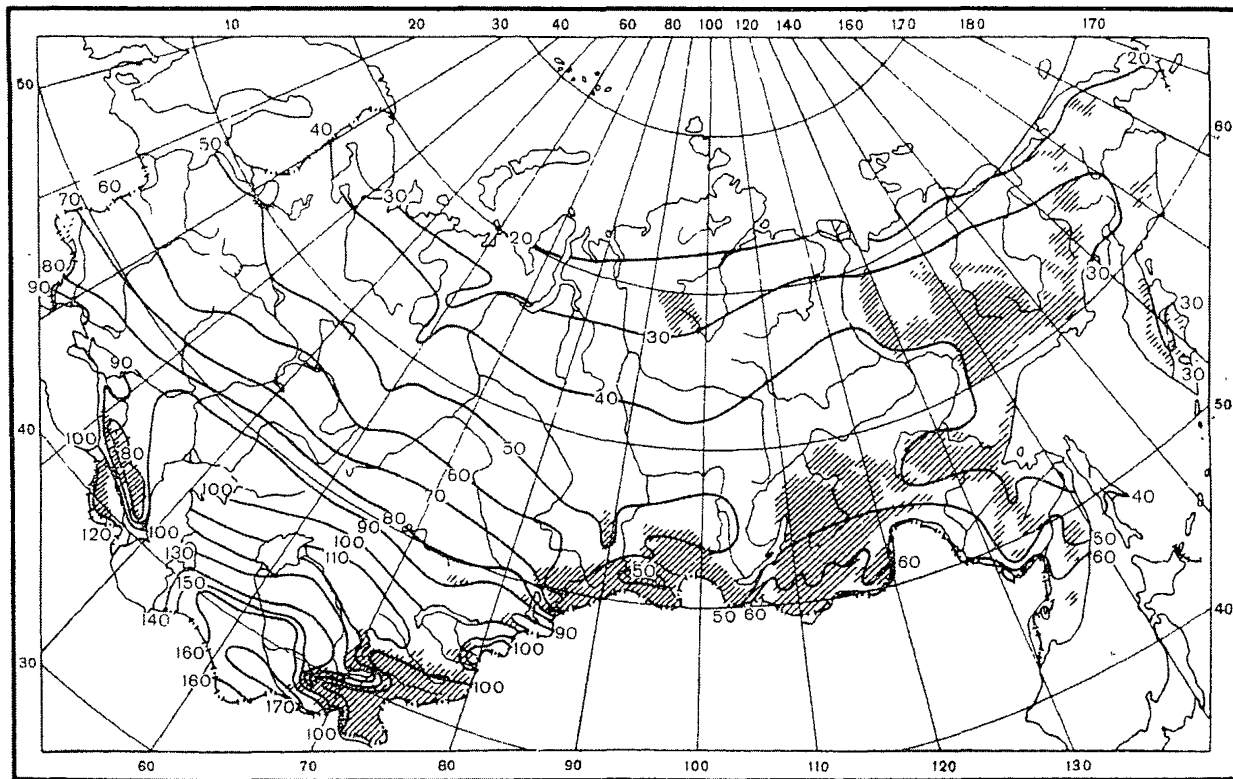
Рис. П2.2. Средняя годовая испаряемость, см ▨ - горные районы
