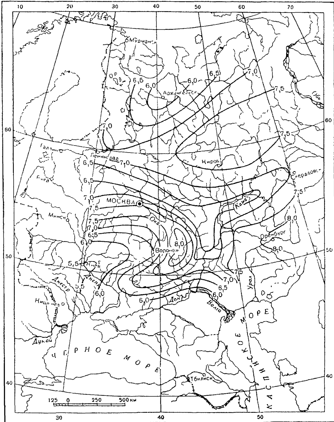
Рис. П2.22. Карта максимальной часовой интенсивности снеготаяния 1%-ной обеспеченности в мм/ч (по П. П. Кузьмину)
