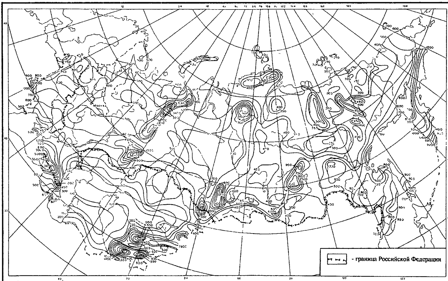
Рис. П2.1. Среднее годовое количество осадков, мм
