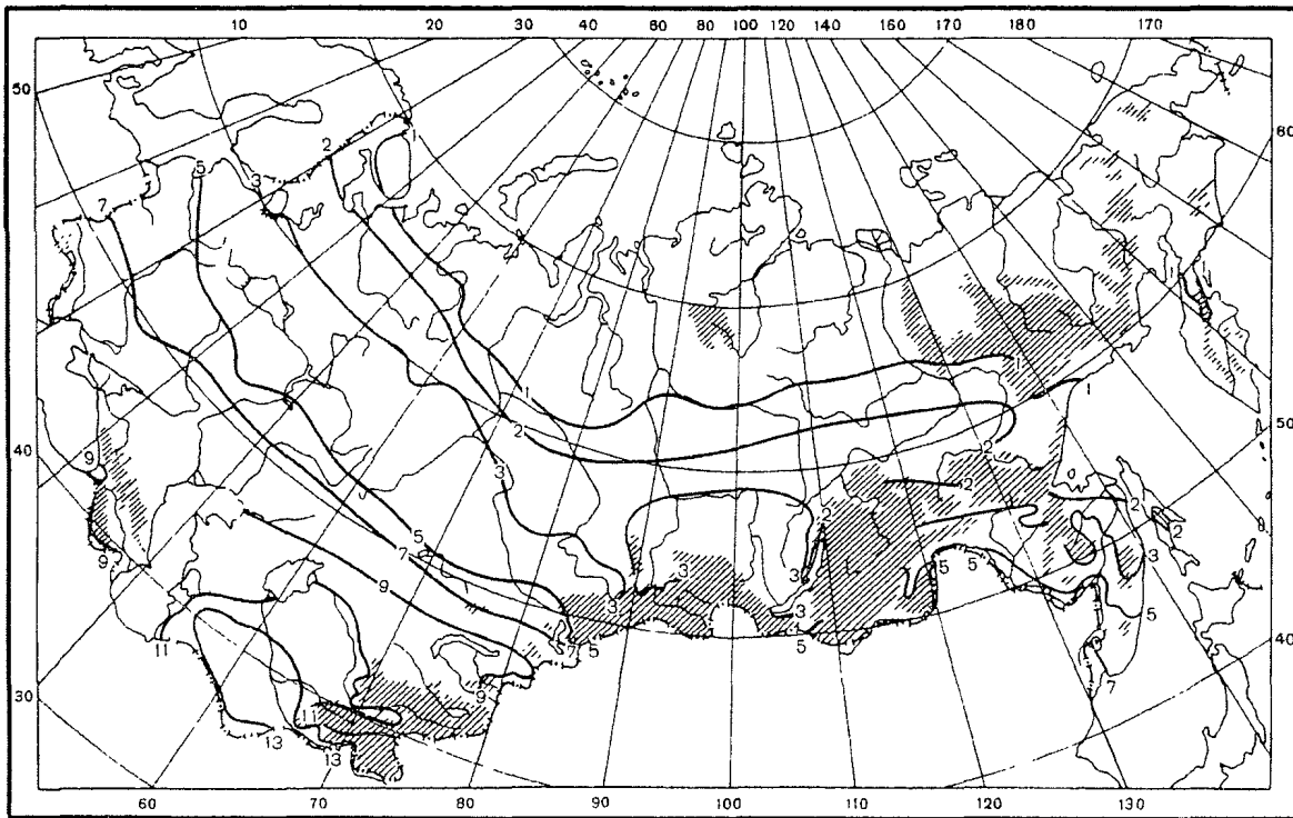
Рис. П2.6. Средняя месячная испаряемость, см. Апрель
