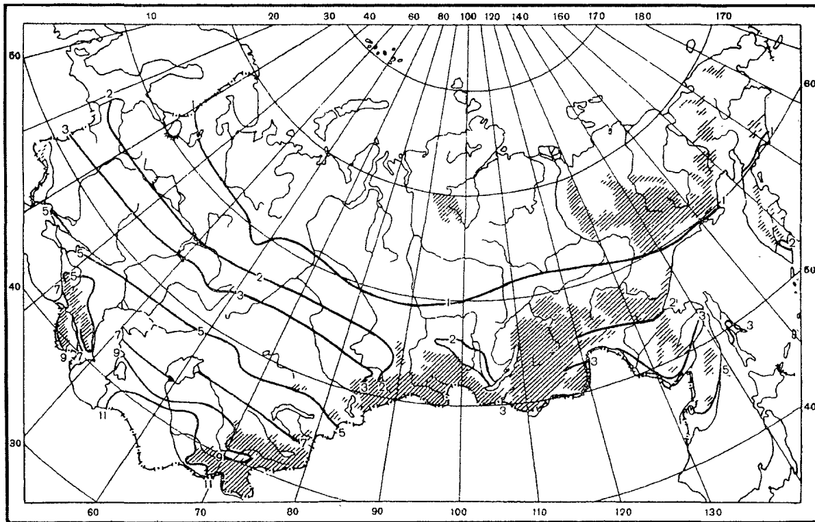
Рис. П2. 12. Средняя месячная испаряемость, см. Октябрь ▨ – горные районы
