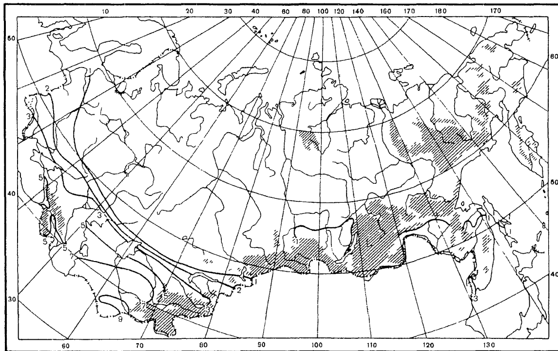
Рис. П2.5. Средняя месячная испаряемость, см. Март
