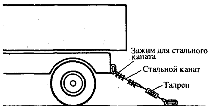
Рис. П.3.2. Крепление автомашины с помощью найтовов из стального каната
