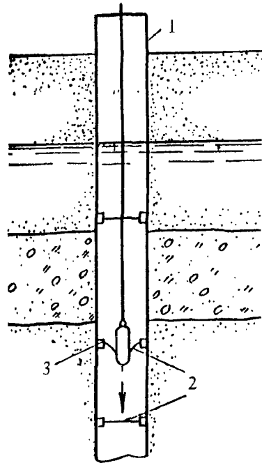
Схема обустройства наблюдательных скважин эластичными лепестковыми диафрагмами для термокаротажа фильтрационных потоков
