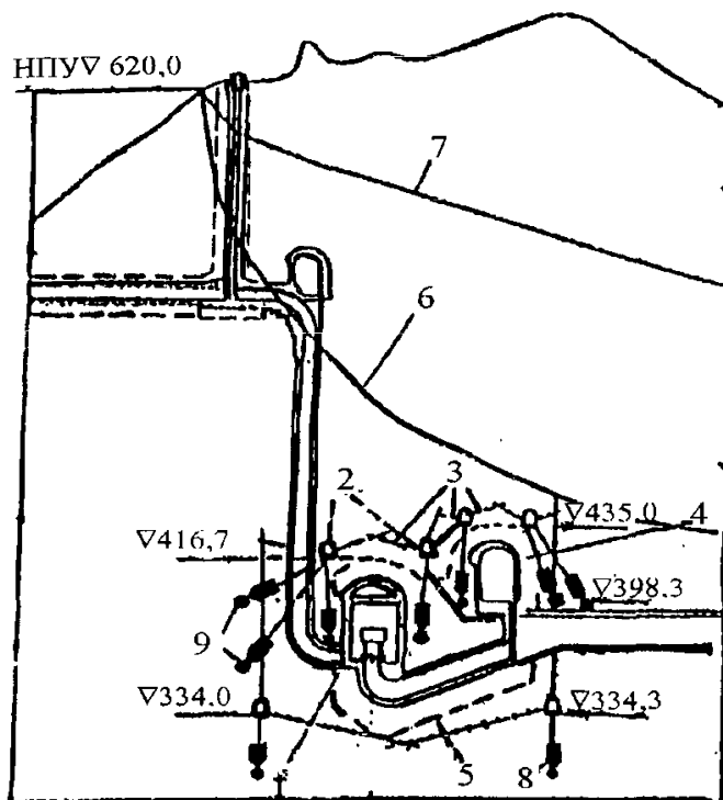
Рис.П.4. Поперечный разрез здания ГЭС
