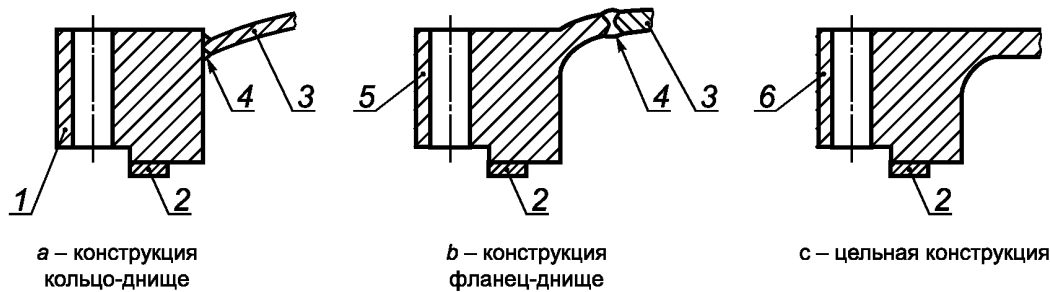
1 — кольцо; 2 — прокладка; 3 — днище; 4 — сварной шов с полным проплавлением; 5 — фланец; 6 — цельная механически обработанная крышка
