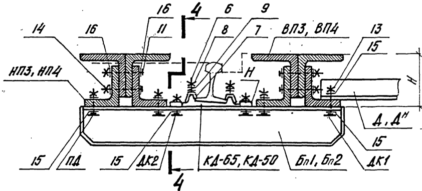
Исполнения 2233 1.0.0.0-03, -04, -05
