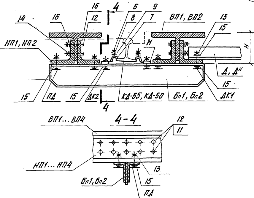
Исполнения 2233 1.0.0.0, -01, -02
