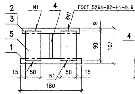
Вид А
