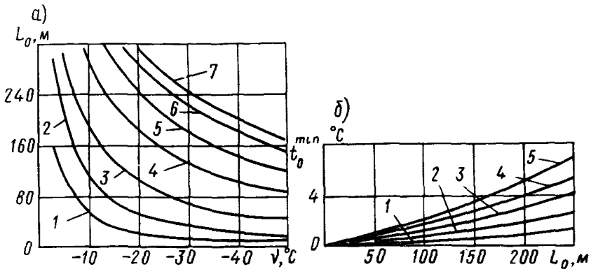
Рис. 44. Зависимость длины пути охлаждения гидросмеси от начальной температуры t_0 до 0^\circ\text{C} для различных значений \psi t_0 = 0,2; 0,5; 1,0; 2,0; 3,0; 4,0; 5,0 (линии 1-7), b_0 = 200 м (а); зависимость минимально допустимой температуры гидросмеси от линии пляжа намыва: \psi = -10, -20, -30, -40, -50^\circ\text{C} (линии 1-5) (б)
