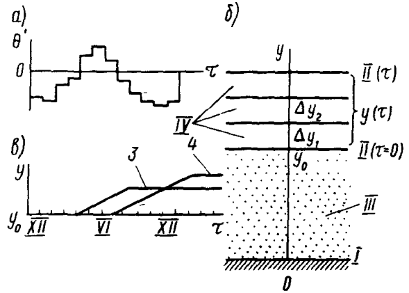
Рис.42. Схема к прогнозу температурного режима дамбы
