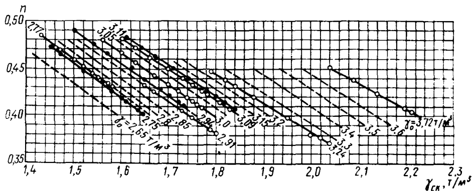
Рис. 4. Зависимость изменения пористости n от плотности сухих отходов \gamma_{ск} при разных значениях плотности частиц отходов \gamma_o
