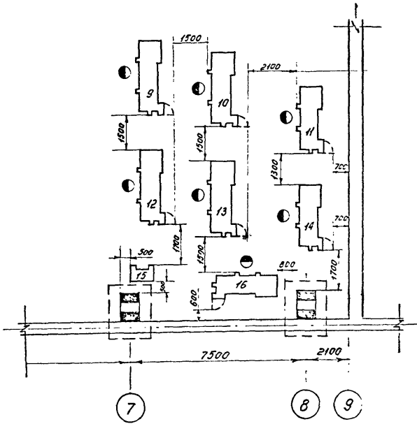
Рис. 3 Пример изображения технологического оборудования и его привязки в проекте и утверждаемой части рабочего проекта
