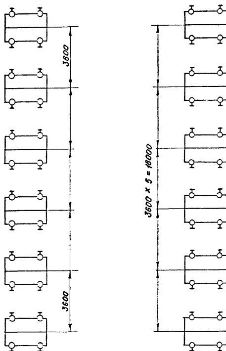
Рис. 1 Пример простановки размеров ряда одинаковых элементов, расположенных на равных расстояниях друг от друга
