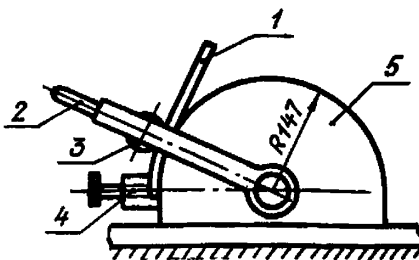
1 - пластина; 2 - ручка; 3 - ролик; 4 - зажим; 5 - барабан
