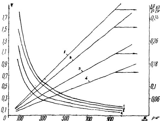
Рис. 8. Значения f и \frac{\Delta P}{w^2} в зависимости от z
