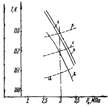
Рис.4. Зависимость производительности трубопровода СПГ ( Q ) и температуры СПГ в конце участка от конечного давления P_k = 2,942 МПа; P_H = 5,393 МПа; T_H = 150 К; K = 0,43 Вт/м 2 ·К
