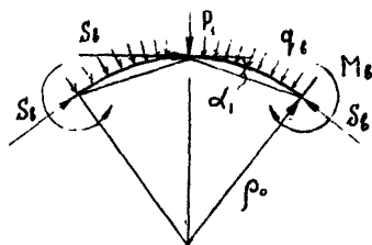
Рис.21. Расчетные схемы постановки крайних условий при распределенной реакции q_B = \frac{S_B}{\rho_0} и при дискретной связи
