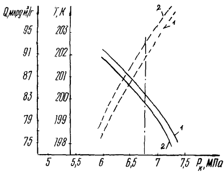
Рис.3. Зависимость производительности трубопровода СПГ ( Q ) и температуры СПГ ( T ) в конце участка от конечного давления P_k = 6,763 МПа; T_H = 9,806 МПа; T_H = 210 К; K = 0,43 Вт/м 2 ·К
