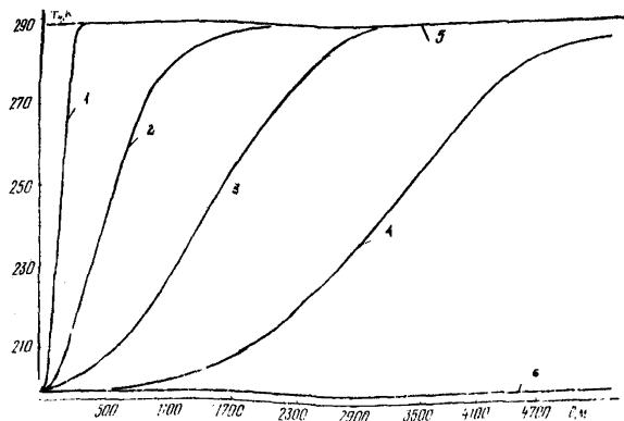
Рис.2. Изменение температуры стенки T_w трубопровода диаметром 1420 мм по длине с T_{вх} = 200 К, массовой скоростью \rho w = 69,15 кг/м 2 ·с:
