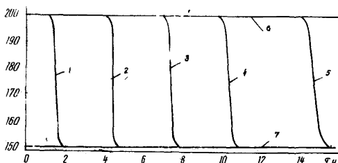
Рис.3. Изменение температуры стенки трубопровода диаметром 1420 мм во времени при захлаживании его от 200 К до 150 К сжиженным при-родным газом (второй этап захлаживания)
