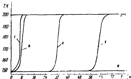
рис.4. изменение температуры стенки трубопровода диаметром 1420 мм по длине при захлаживании его от 200 К до 150 К (второй этап захлаживания):
