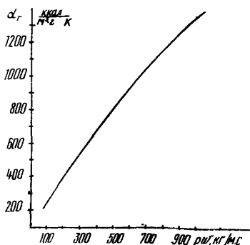
Рис.6. Значения \alpha_r в зависимости от массовой скорости (\rho w) в процессе захолаживания участка трубопровода диаметром 1420 мм
