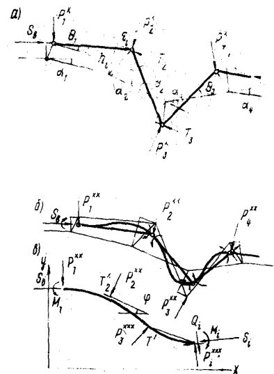
Рис.19. Схема расчета на изгиб:
