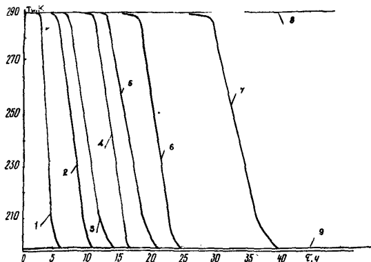
Рис.1. Изменение температуры стенки трубопровода диаметром 1420 мм во времени при захлаживании его газовым потоком с T_{вх} = 200 К, массовой скоростью \rho w = 69,15 кг/м 2 ·с:
