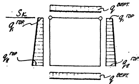
РАСЧЕТНАЯ СХЕМА ТОННЕЛЯ
