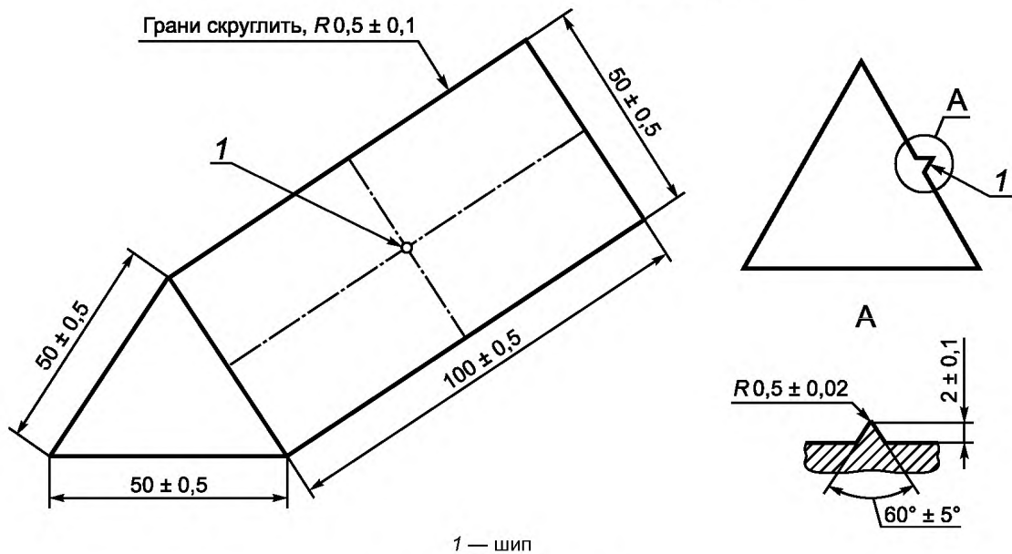
Рисунок 14 — Оправка
