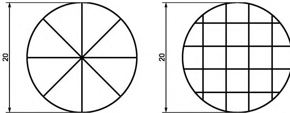
Рисунок 12 — Образец царапин для испытаний на взрывоопасность (см. 18.2.2)
