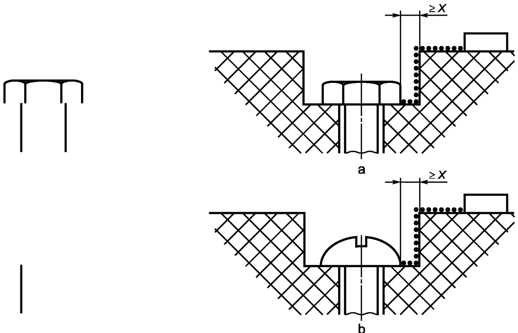
Рисунок Е.8 — Промежуточная, несоединенная проводящая часть
