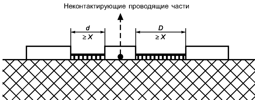
Рисунок Е.7 — Несплошной стык с узкой и широкой канавками
