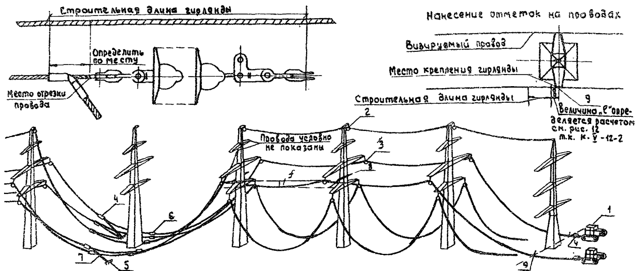
Рис. 5 Натягивание и визуирование проводов на участке ВЛ, ограниченном промежуточной и анкерно-угловой опорами.
