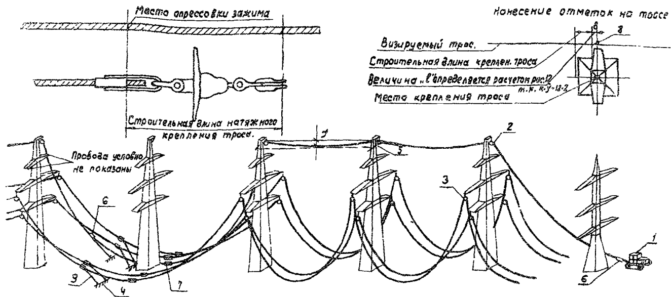
Рис. 4. Натягивание и визирирование грозозащитного троса на участке ВЛ, ограниченном промежуточной и анкерно-угловой опорами.
