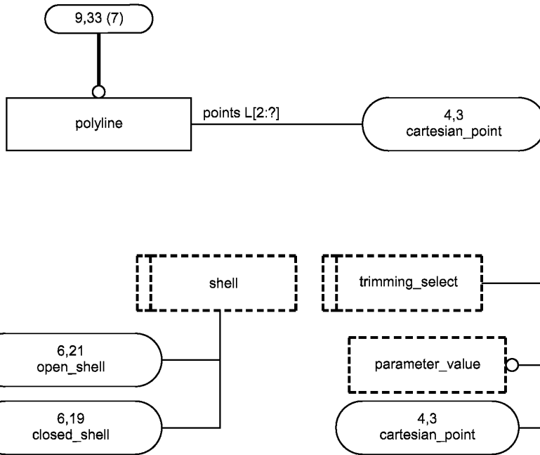
Рисунок С.9 — ПИК manifold_surface_shape_representation в формате EXPRESS-G (диаграмма 9 из 22)
