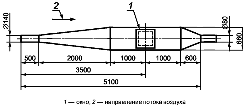
Рисунок 2 — Размеры рекомендуемой испытательной пылевой камеры
