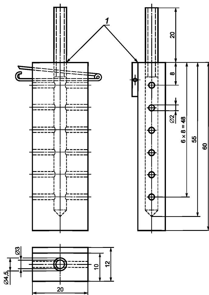
Рисунок 3 — Пробоотборник
