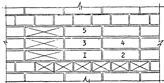
Рис.17. Схемы отбора образцов кирпича и раствора из массива кладки стен а-при чередовании тычек-ложок; б-при трехрядном и более расположении ложков Цифры указывают порядок отбора
