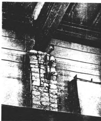
Рис. I3 Вертикальная трещина в кирпичной пилястре.
