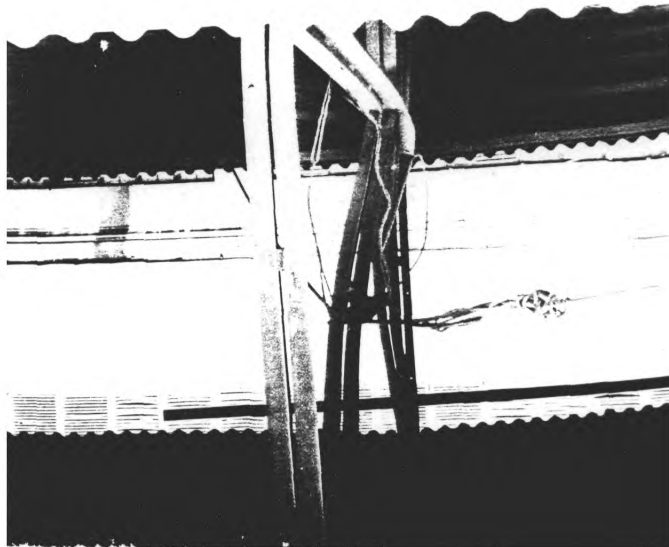
Рис. 5 Деформация верхнего пояса и расколов из плоскости в сварной ферме.
