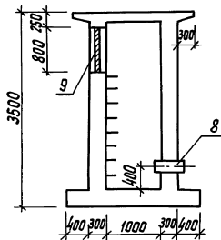
Разрез 2-2
