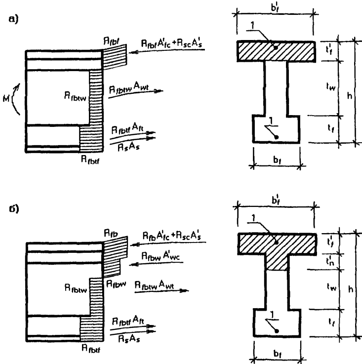
Рис. 4. Схема распределения усилий и эпюра напряжений в сечениях, нормальных к продольной оси изгибаемого элемента двутаврового сечения при комбинированном армировании а – при x \leq t'_f ; б – при x > t'_f ; 1 – стержневая или проволочная арматура.
