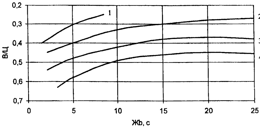
Рис. 1. Графики для подбора отношения Ц:П, обеспечивающего требуемую жесткость сталефибробетонной смеси в зависимости: а — от жесткости исходного бетона при \mu_{fv} : 1 — 1%; 2 — 1,5%; 3 — 2,5%. б — цементно-песчаного отношения Ц:П от жесткости исходного бетона Жб и водоцементного отношения Ц:П равного: 1 — 1:1; 2 — 1:2; 3 — 1:3; 4 — 1:4.
