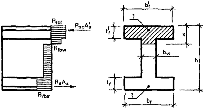
Рис. 1. Схема внутренних усилий и эпюры напряжений в сечении, нормальном к продольной оси элемента (общий случай) 1 – сосредоточенная стержневая или проволочная арматура
