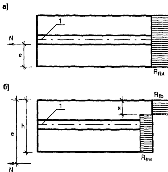
Рис. 7. Эпюры напряжений во внецентренно растянутых элементах прямоугольного сечения а – при приложении продольной силы N в пределах ядра сечения; б – то же, за пределами; 1 – стержневая или проволочная арматура.
