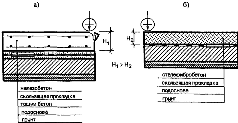
Рис. 1.Ж. Сопоставительные конструктивные решения промышленных полов по грунтам: а) традиционный железобетонный пол; б) сталефибробетонный пол.
