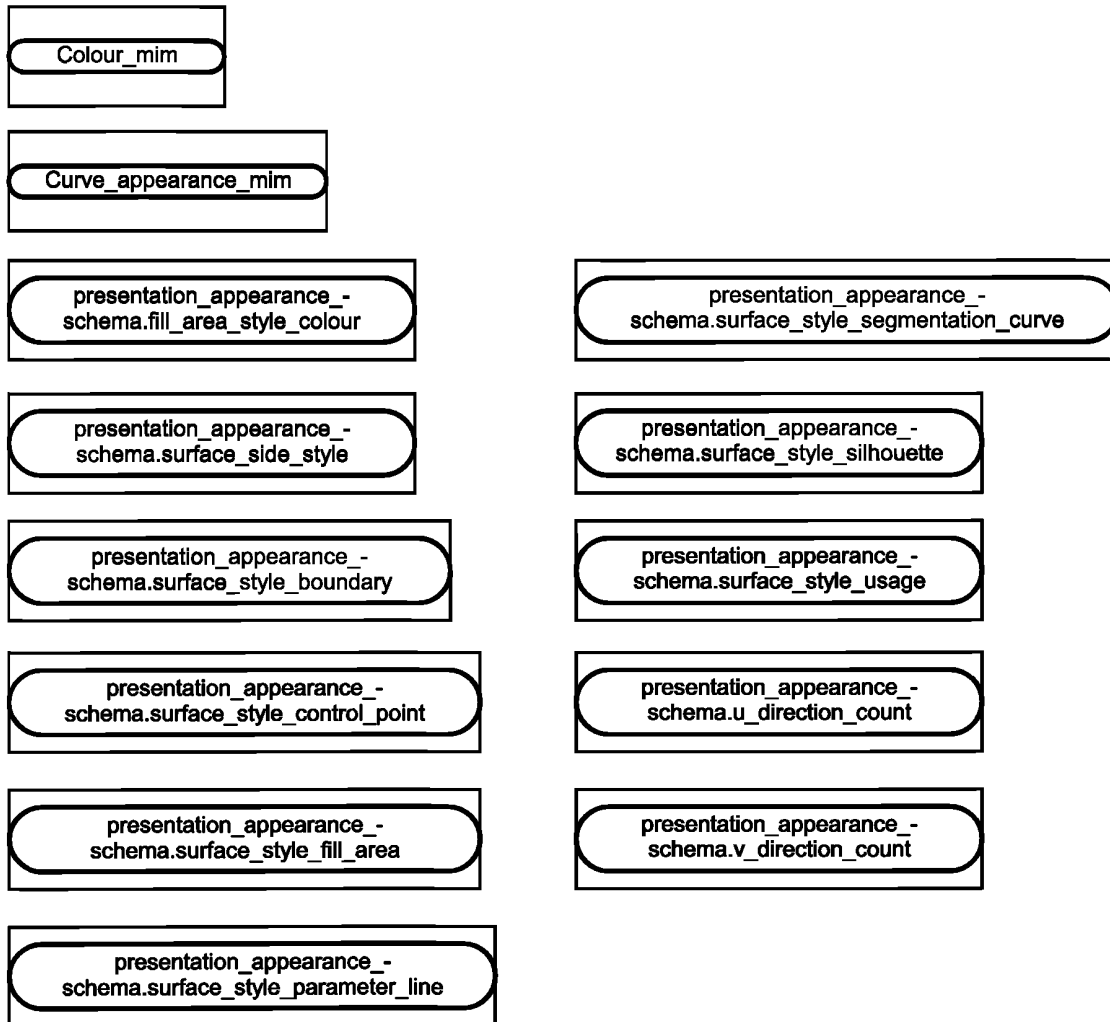
Схема D.1 — EXPRESS-G диаграмма IMM
