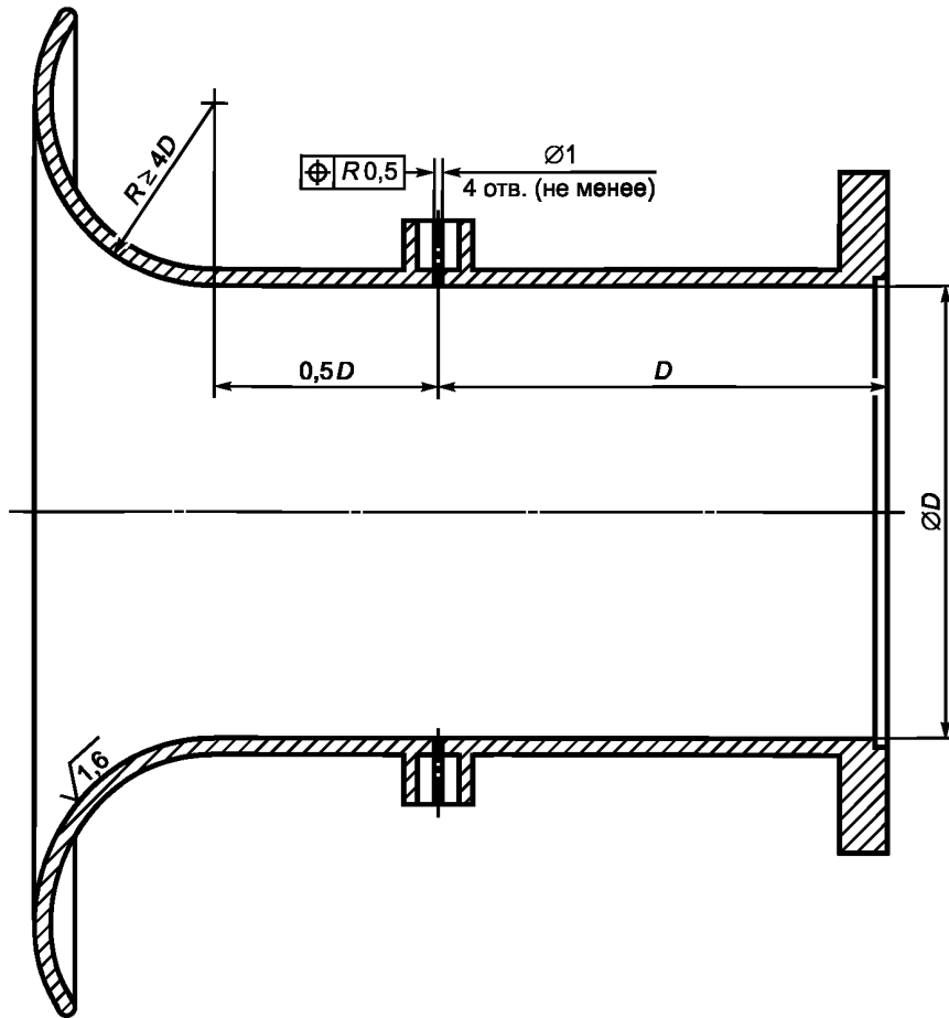
Рисунок 1 — Коллектор для измерения расхода воздуха
