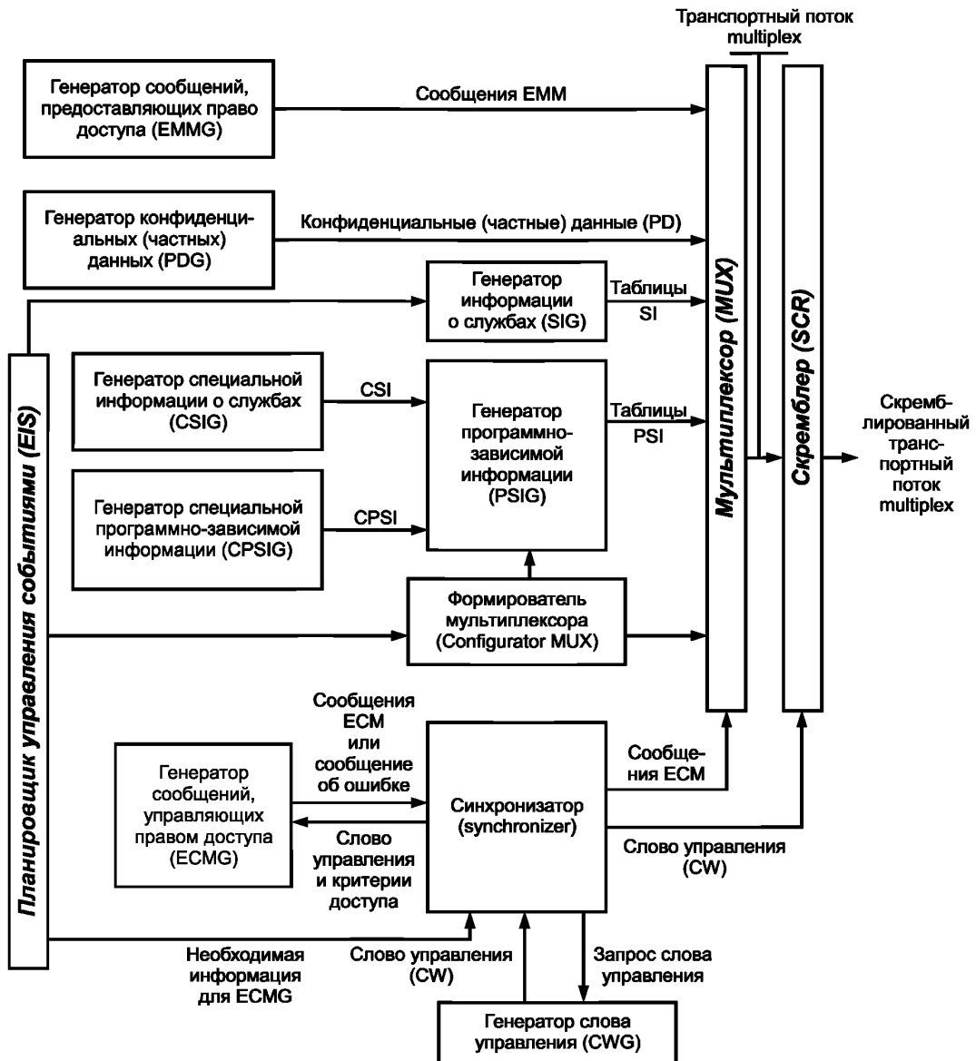
Рисунок 5 — Структурная схема передающей части оборудования СОД Multicrypt
