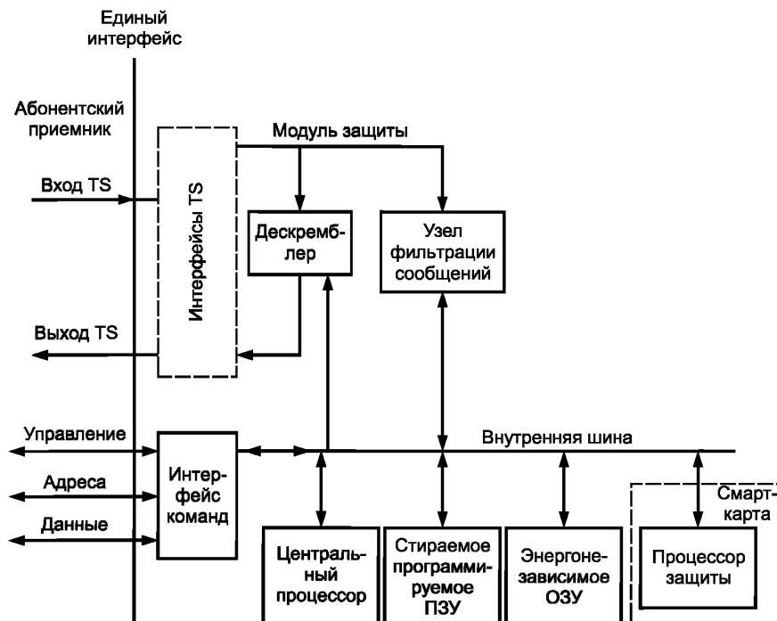
Рисунок 7 — Структурная схема модуля защиты
