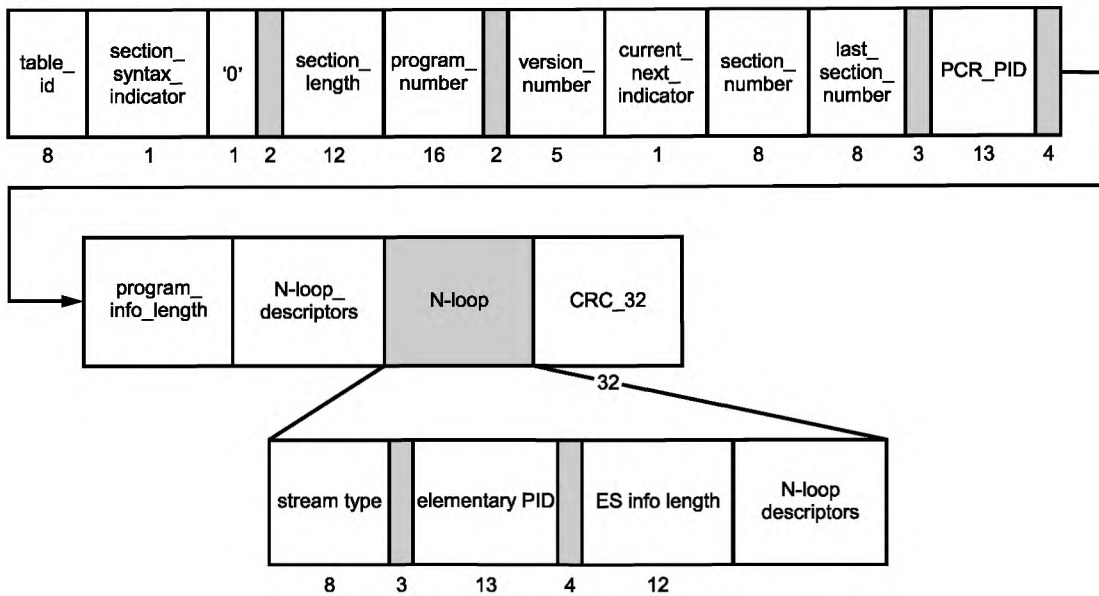
Рисунок А.5 — Структура полей секции таблицы PMT
