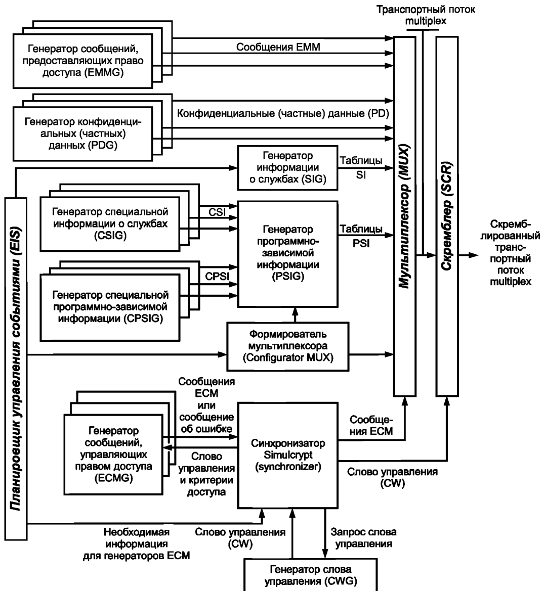
Рисунок 4 — Структурная схема передающей части оборудования СОД Simulcrypt
