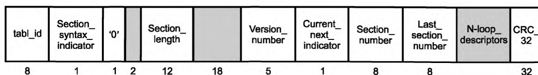
Рисунок А.4 — Структура полей секции таблицы CAT
