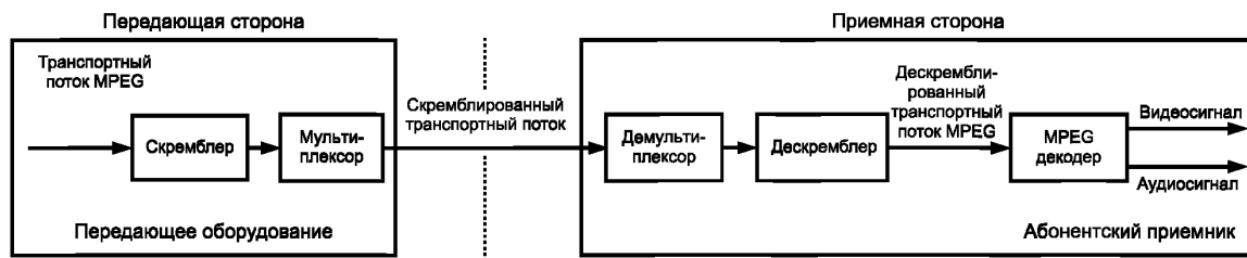
Рисунок 1 — Структурная схема одноуровневой СОД
