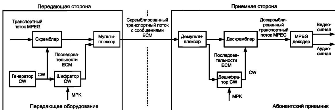
Рисунок 2 — Структурная схема двухуровневой СОД
