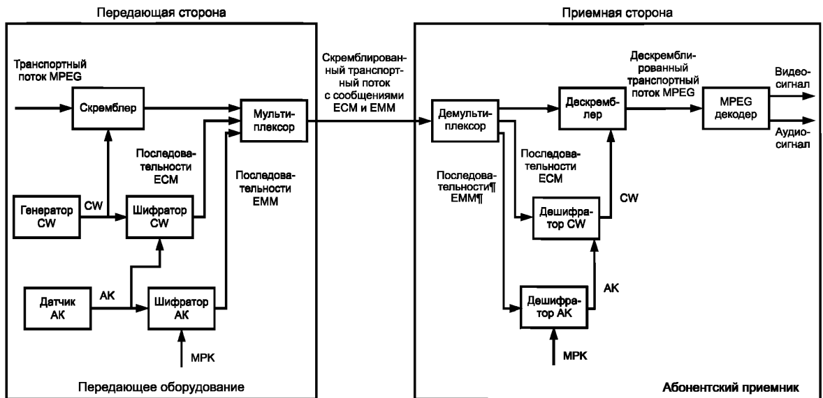
Рисунок 3 — Структурная схема трехуровневой СОД
