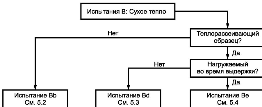
Рисунок 1 — Блок-схема испытаний V: Сухое тепло
