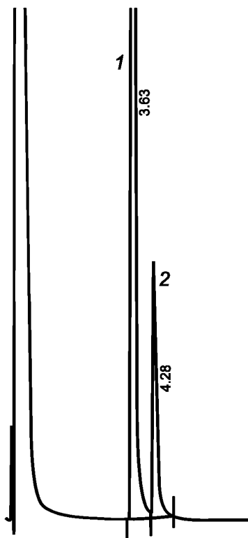
1 — 1,4-бутандиол; 2 — глицерин
