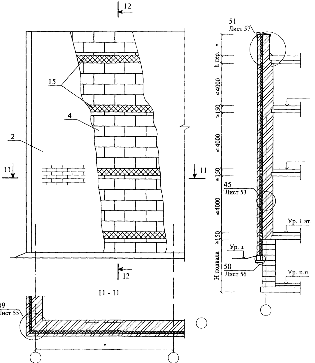
СХЕМА № 8. Расположение плит утеплителя, рассечек
