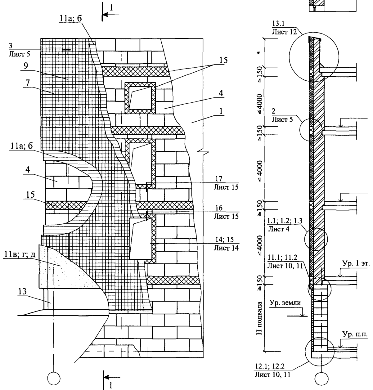
СХЕМА № 1. Расположение плит утеплителя, рассечек, сетки и штукатурки
