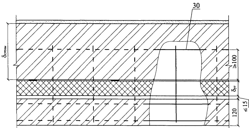
1. Узлы 39; 40 - возможные варианты соединения слоев кладки
