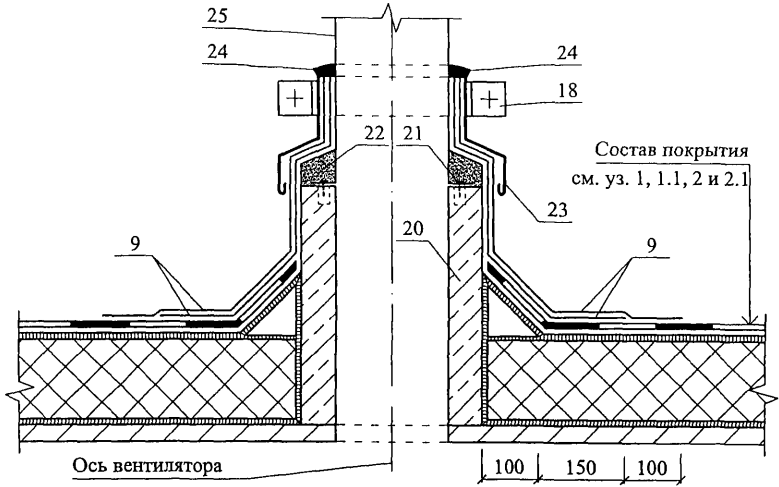
7 Пропуск трубы через покрытие
