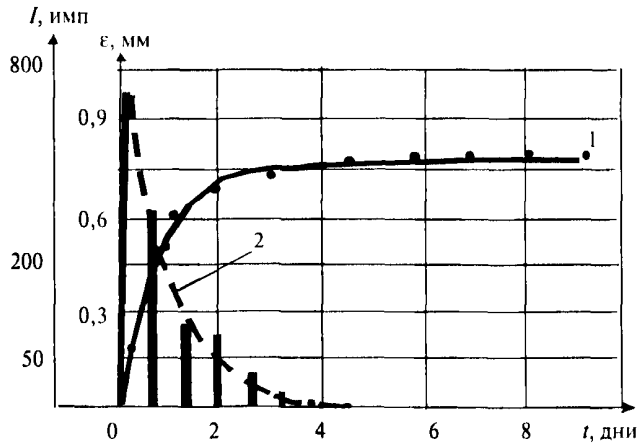
Рисунок 3.6 — Изменение деформаций ( I ) и сигналов АЭ ( 2 ) после разгрузки песчано-цементного образца, сформированного под давлением на скелет, равным 10 МПа
