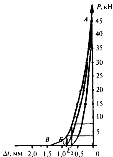
Рисунок Б.3 — Экспериментальные результаты разгрузки образцов с различной прочностью цементирующего раствора: AE_1 и AE_2 — составов 6:1 и 3:1 (песок : цемент); AB — с незатвердевшим («сырым») раствором
