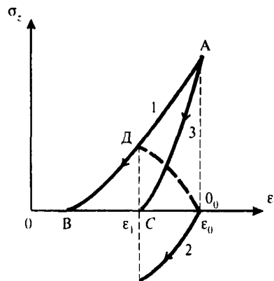
Рисунок Д.1 — График совмещения зависимостей между напряжениями и деформациями при разгрузке для элементов, слагающих породу
