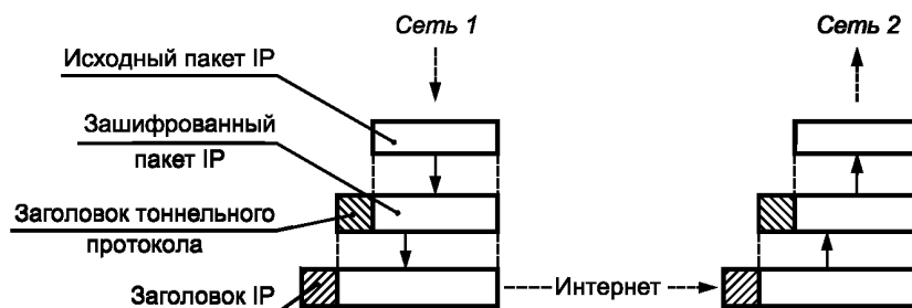
Рисунок 3 — Инкапсуляция IP-пакетов
