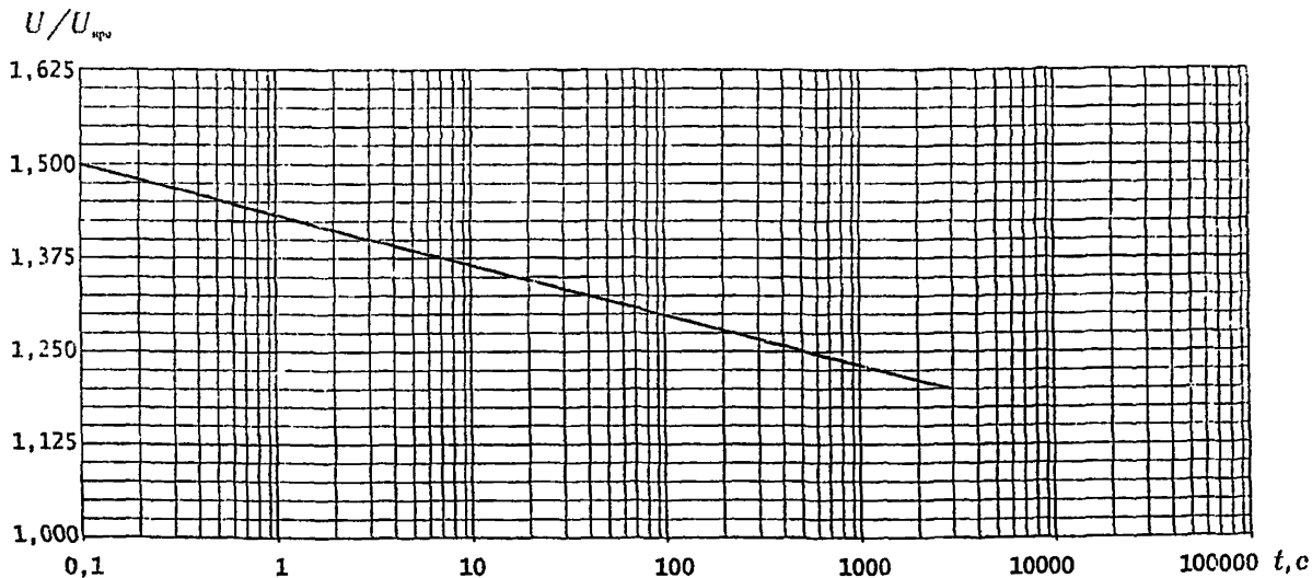
Рис.7. Зависимость "допустимое напряжение-время" для случая предварительного нагружения импульсом 2,25 \text{ кДж/кВ } U_{нр} для ОПН, выпускаемых ООО "Таврида-Электрик" по ТУ № ИТБА 674361.0005.
