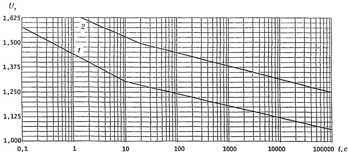
Рис.5. Зависимость "допустимое напряжение-время" для случая без предварительного нагружения импульсом энергии для ОПН, выпускаемых АООТ "КФЗ" по ТУ №: 1) 3414-019-04682628-97, 2) 3114-011-04682628-96.
