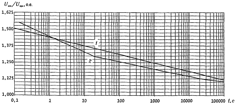
Рис.6. Зависимость "допустимое напряжение-время" для случая:
