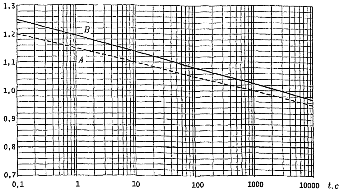
Рис.1. Зависимость относительных величин временных перенапряжений U , промышленной частоты, которые должны выдерживать ОПН EXLIM R, от их длительности.
