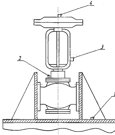
а) вертикальное положение оси клапана по отношению к платформе
