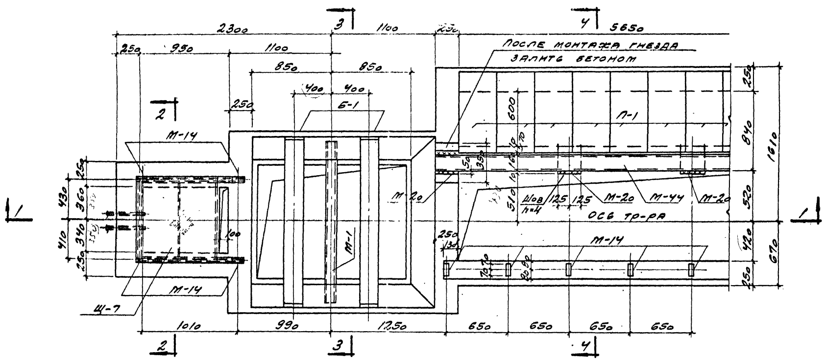
ЭЛЕМЕНТ ПЛАНА 1
